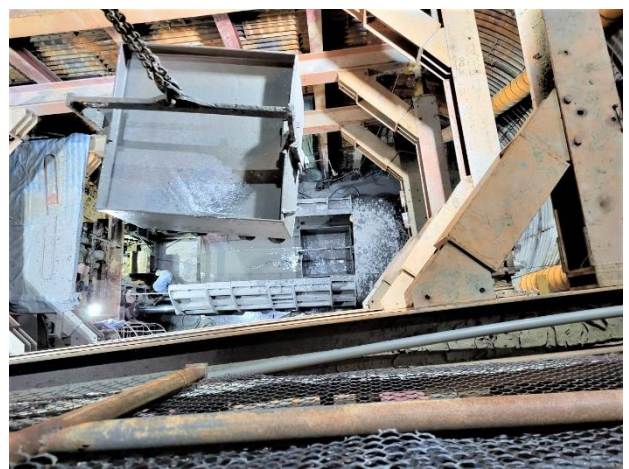
W57 工作井：推進工程施作
