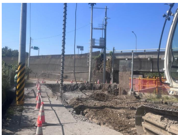
W59 工作井 → 終點： 銜接 IV-11 球閥 鋼軌樁引孔
