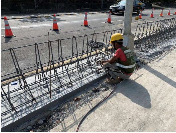
W39 工作井 → 中正段： 中央分隔島施作
