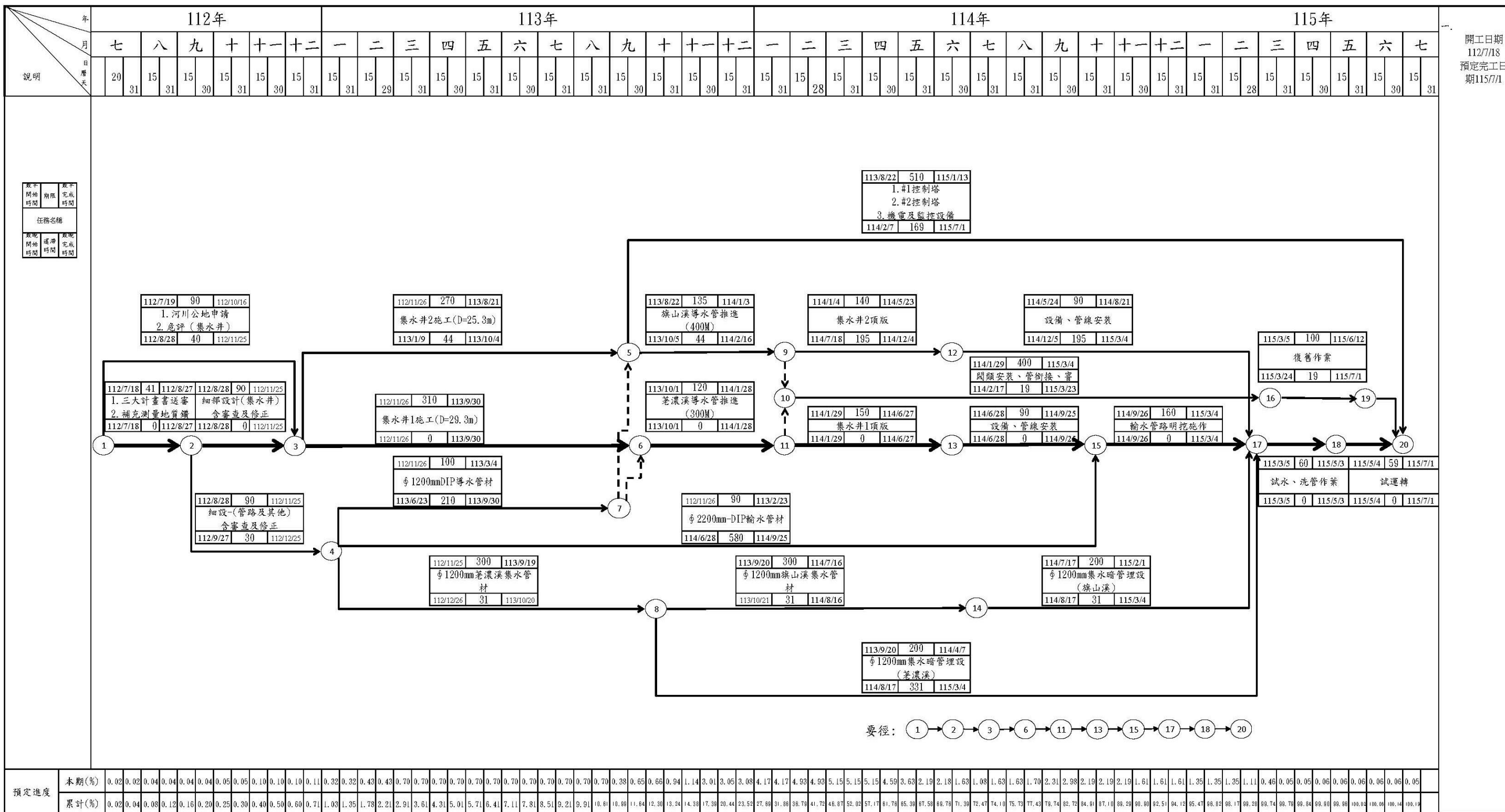
老濃溪(里嶺)伏流水統包工程—網狀圖
