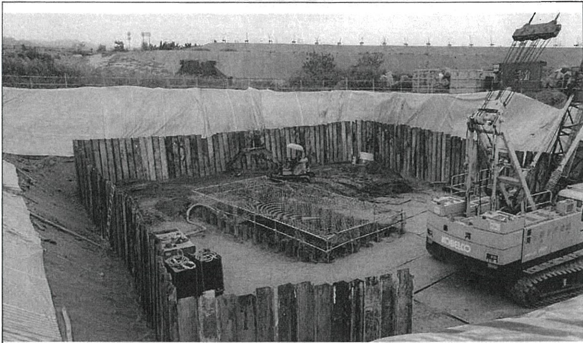
集水井#1 周邊施工現況-1
