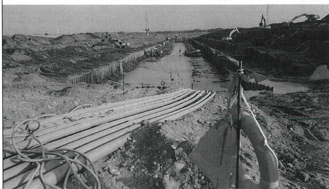
集水井#1 周邊施工現況-2
