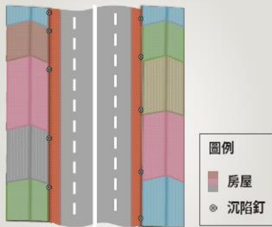
沉陷釘設置俯視示意圖
