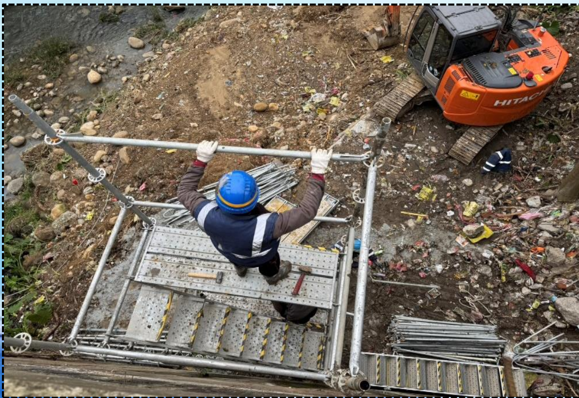
關西二號橋A1橋台上下設備搭設
