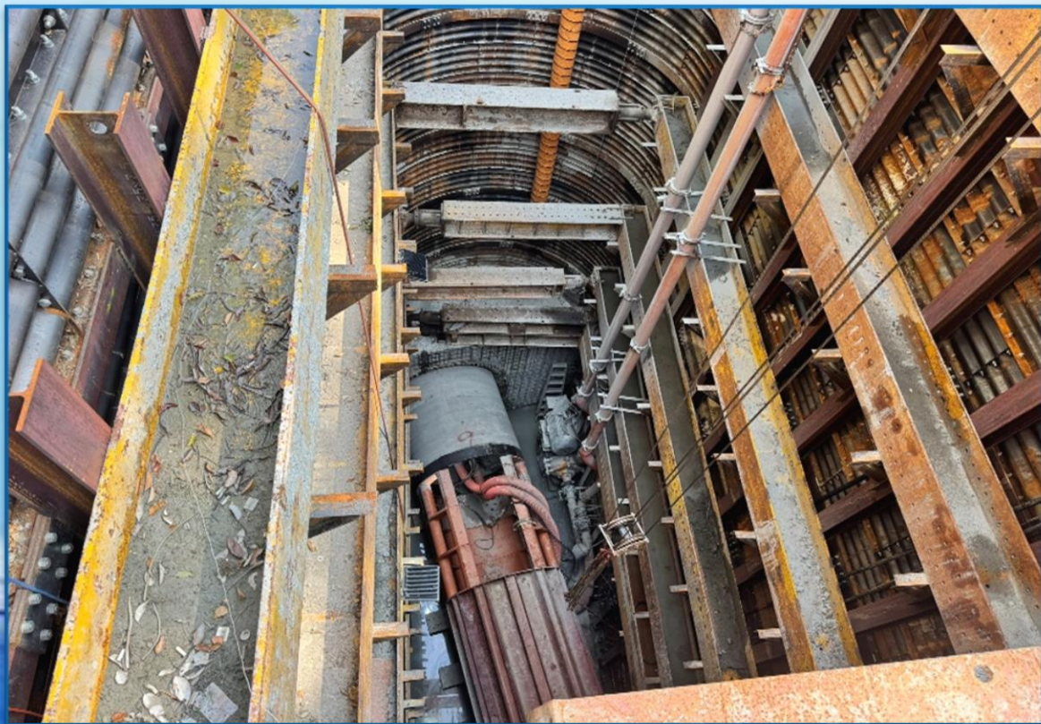
W02→W01推進作業
