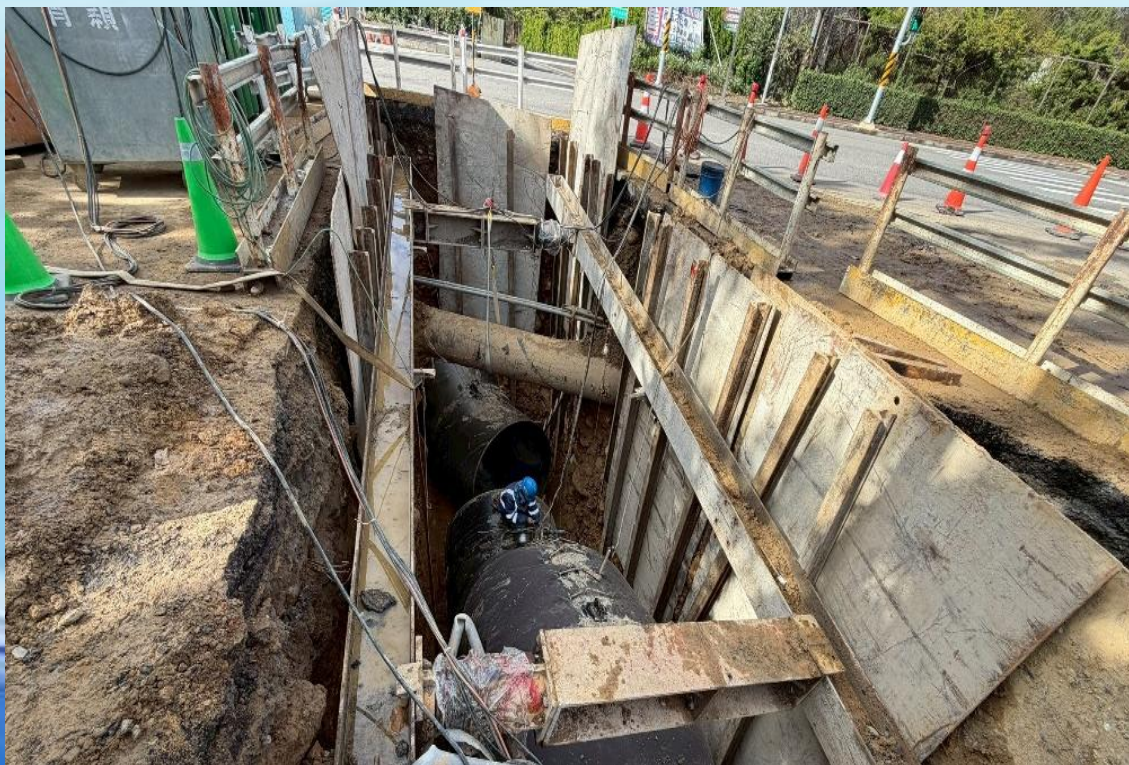
竹28-1銜接段SP鋼管焊接作業
