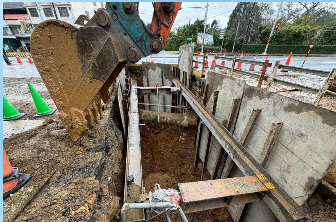
竹28-1銜接段既有管線附掛
