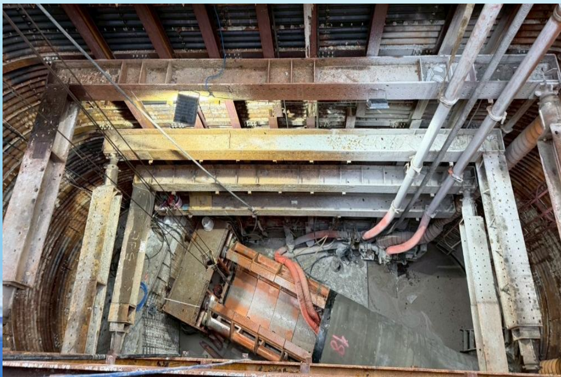
W03→W04推進作業
