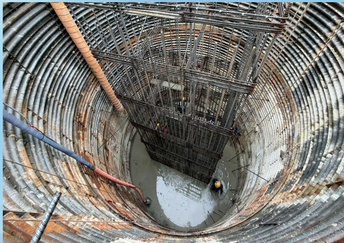
北沙坑橋A1橋台鋼筋綁紮
