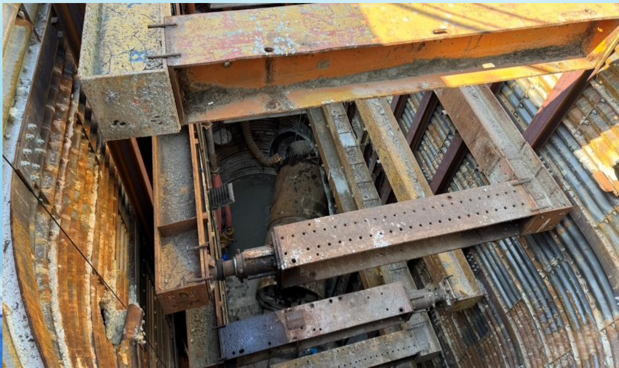
W03→W04推進作業
