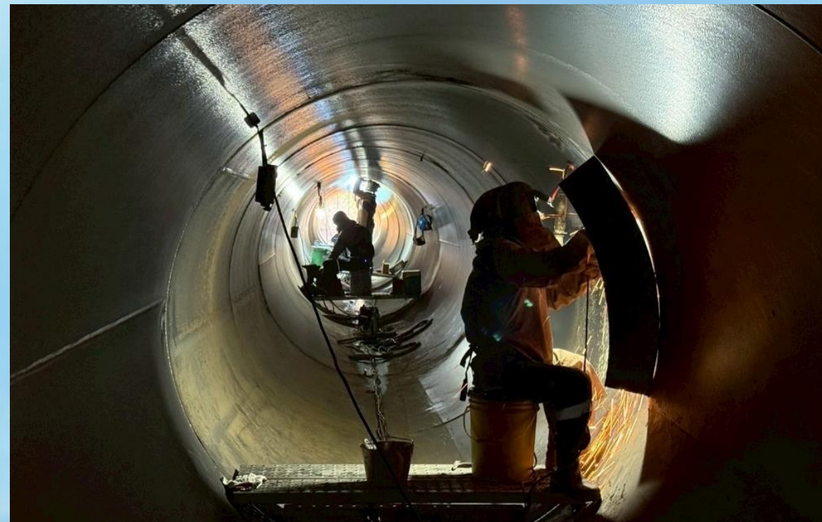
第二工區焊接作業
