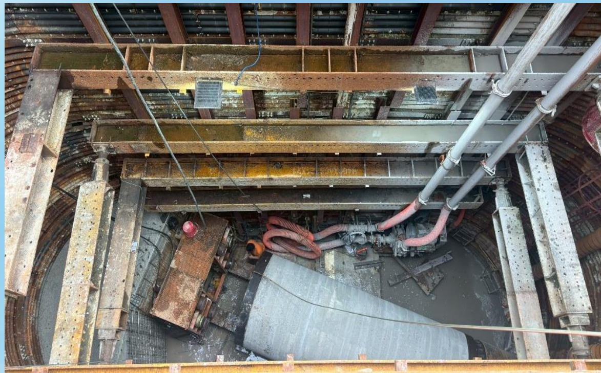
W03→W04推進作業
