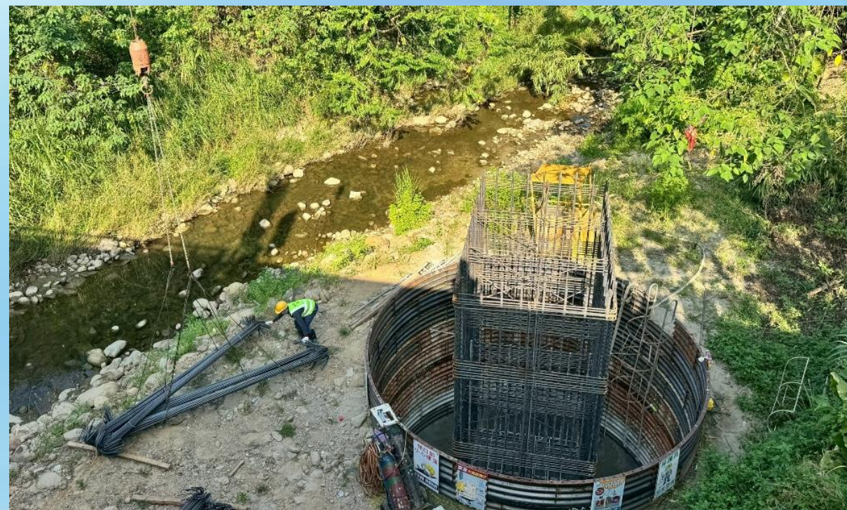
關西二號橋A1橋台鋼筋綁紮
