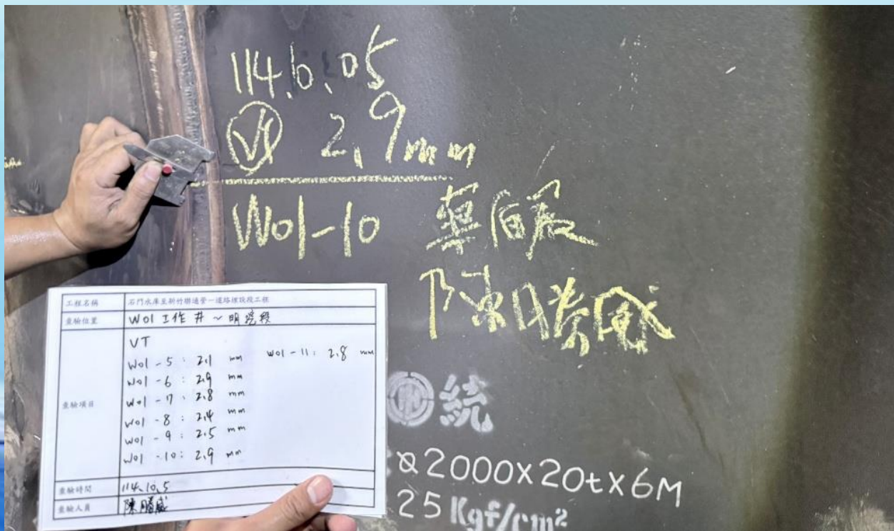
第二工區非破壞檢驗
