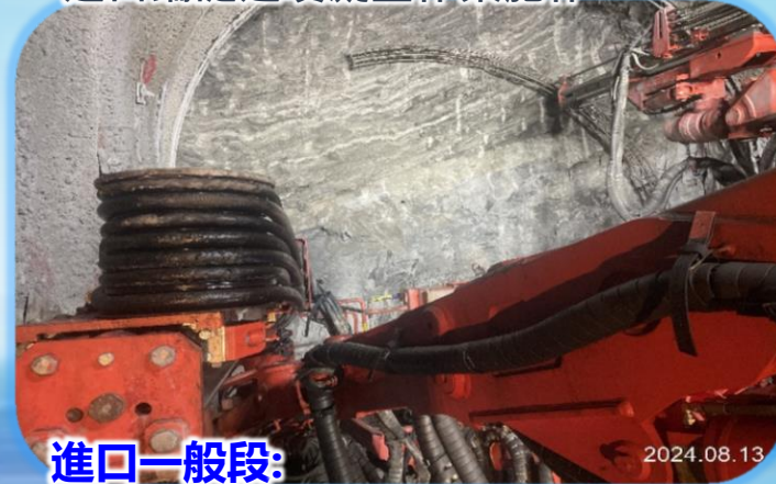
進口一般段： 進口端隧道噴凝土作業施作。
