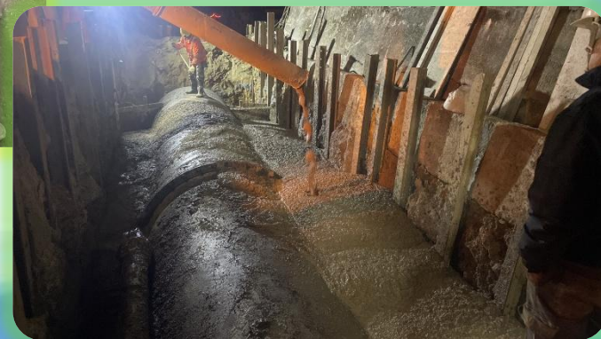
明挖段: CLSM澆置作業
