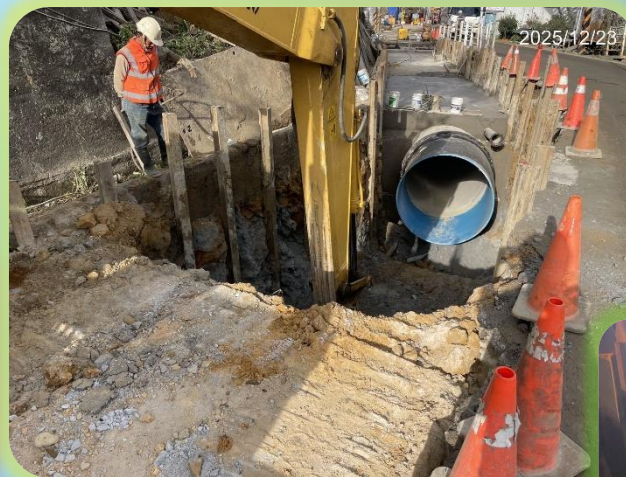
明挖段: 開挖作業
