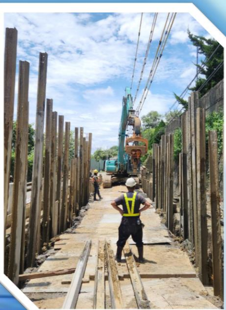
明挖段: 鋼軌樁拔除。
