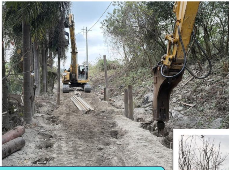
第三工區 鋼軌樁打設
