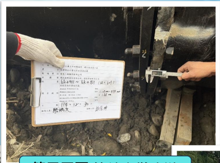
第二工區 管線安裝查驗
