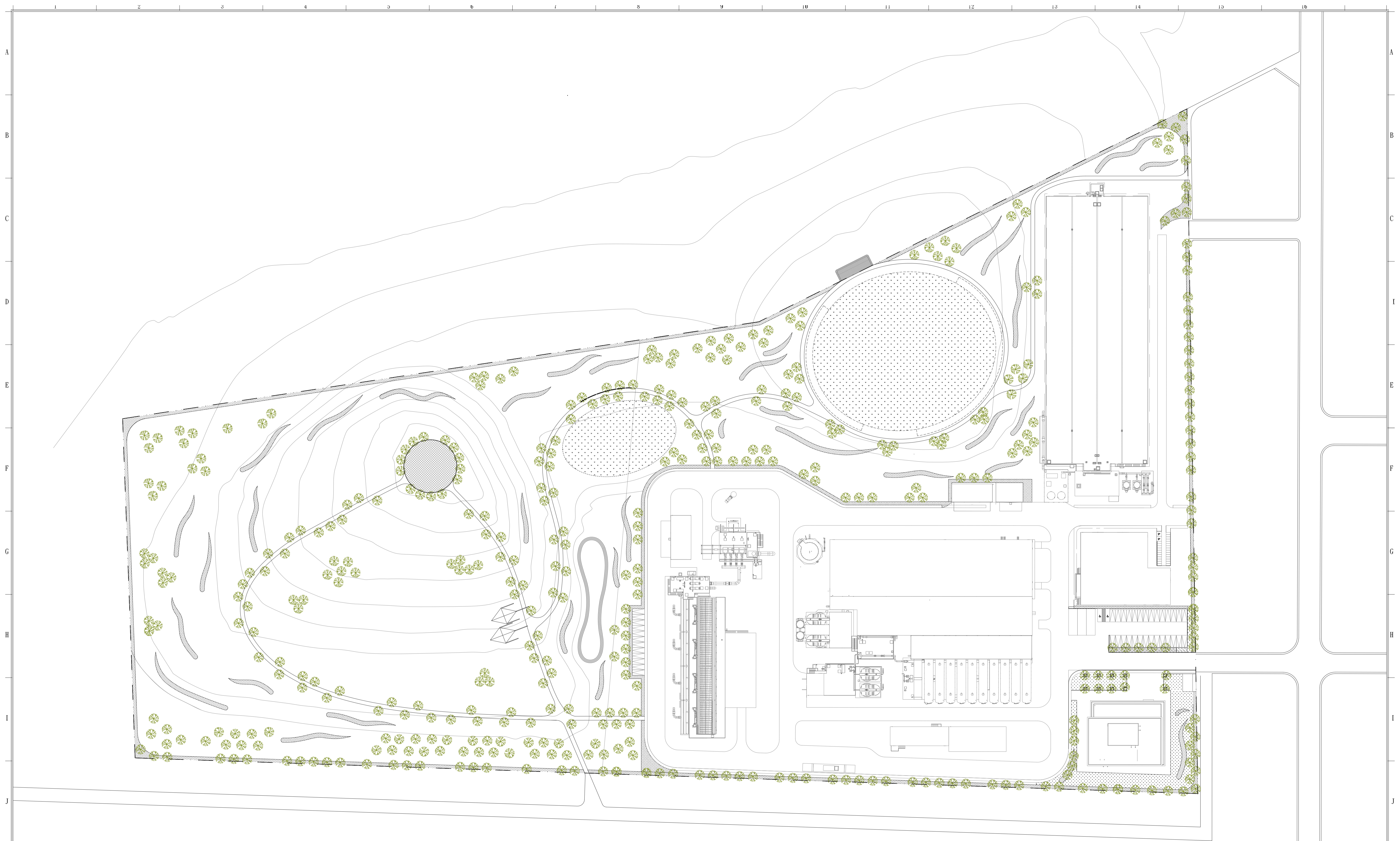
01 景觀平面圖 SCALE: A1:1/750 A3:1/1500 UNIT: cm
