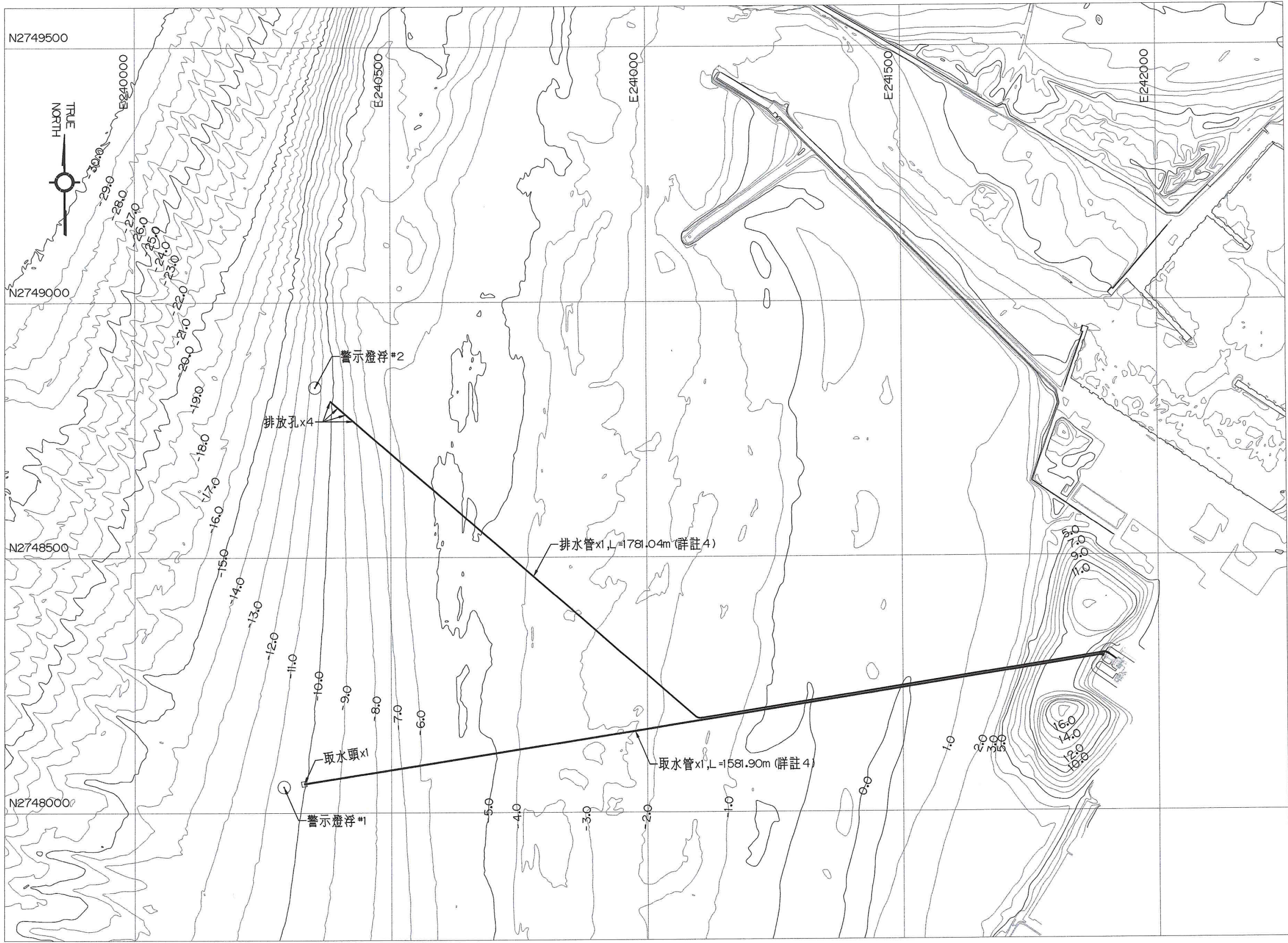
取排水管線總平面圖 A1:1/4000, A3:1/8000
