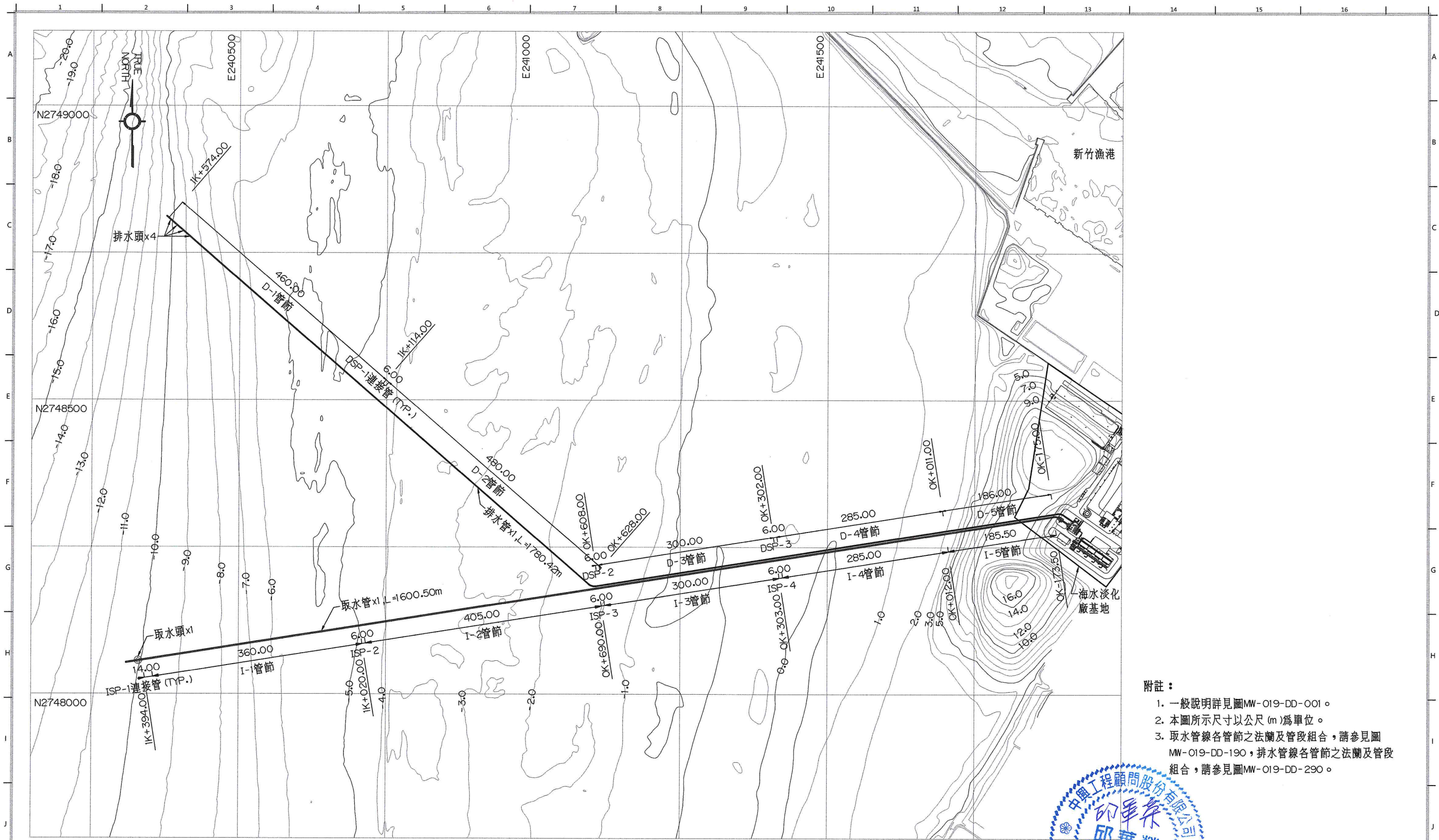
取排水管線管節平面圖 A1-1: 3000, A3-1: 6000
