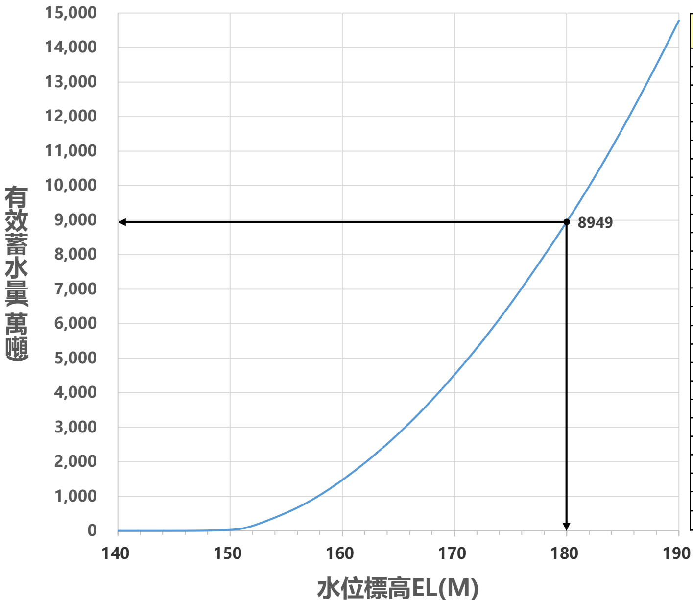
南化水庫水位-蓄水量對照圖
