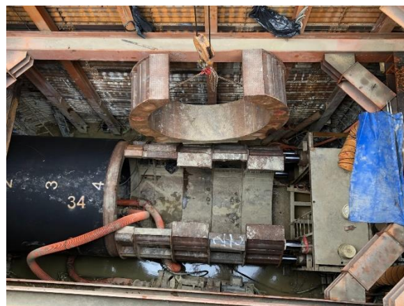
W41 工作井：推進工程施作
