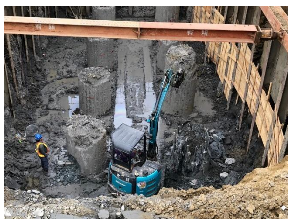
鏡面水庫水管橋：A2 橋台 樁頭打除
