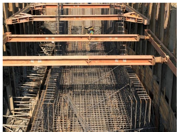
鏡面水庫水管橋：A2 橋台 基礎鋼筋綁紮
