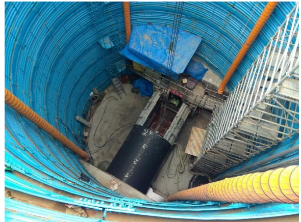
W59 工作井：推進工程施作
