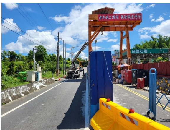
W57 工作井：推進設備安裝
