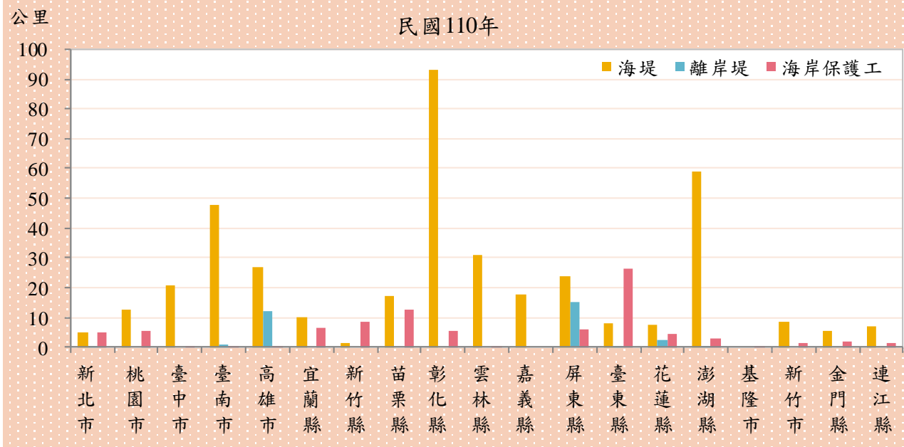
圖 12 現有禦潮(海堤)設施--海堤、離岸堤、海岸保護工
