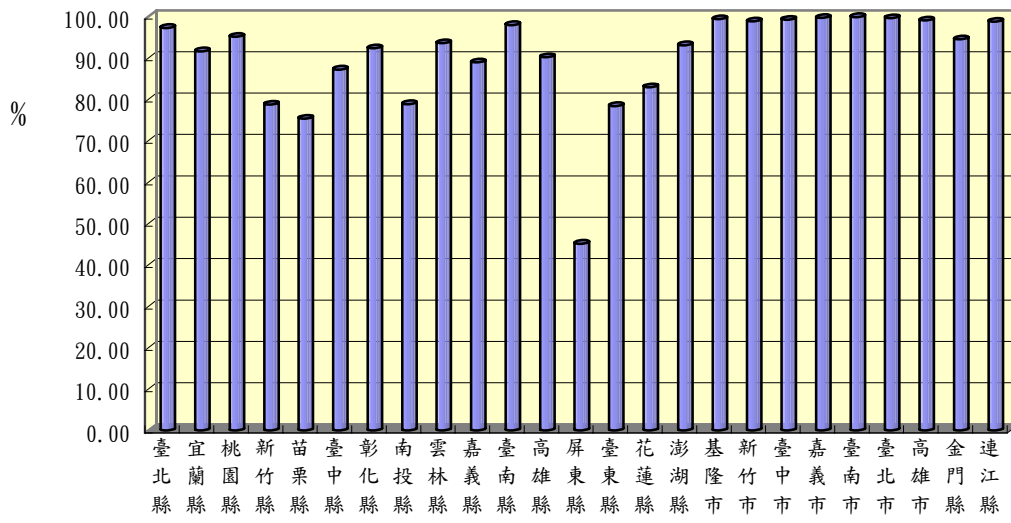
各縣市自來水供水普及率比較圖 民國97年12月底
