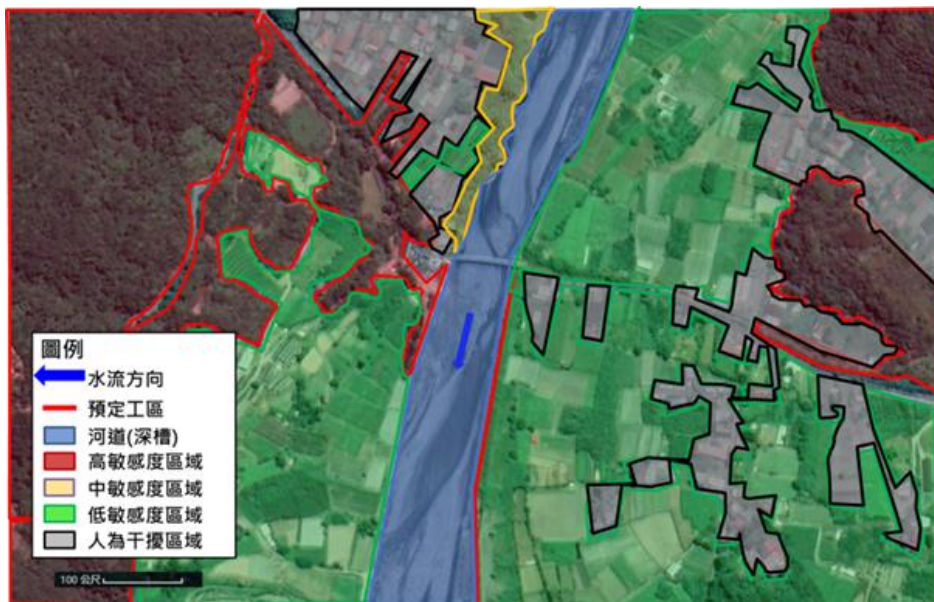
圖 4-127 濁水溪新武界橋下游左岸堤段(0+000~0+600)整建工程生態關注圖
