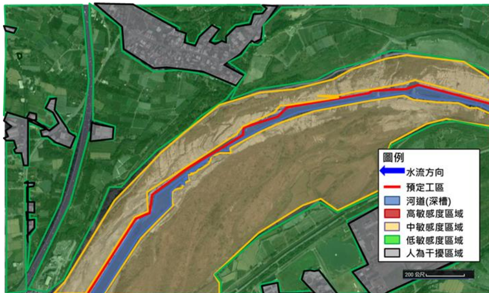
圖 4-135 濁水溪濁水、社寮、富州等堤防(斷面 105~114)整建工程生態關注圖
