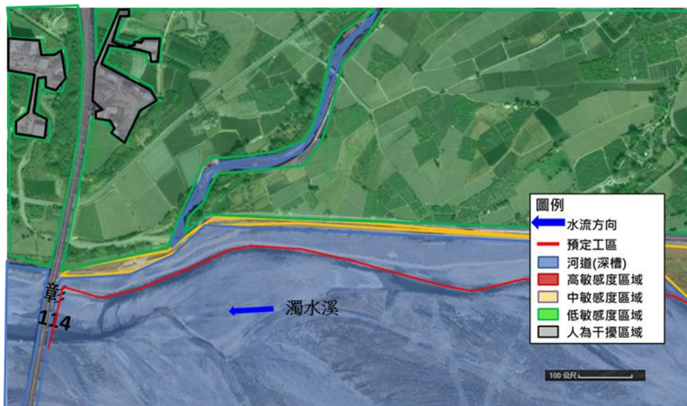
圖 4-133 濁水溪濁水低水護岸(斷面 87~105)整建工程生態關注圖
