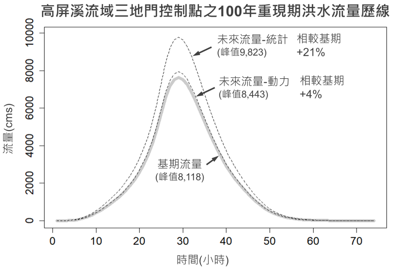
圖 5-2 高屏溪流域三地門控制點於氣候變遷影響下之洪水流量歷線
