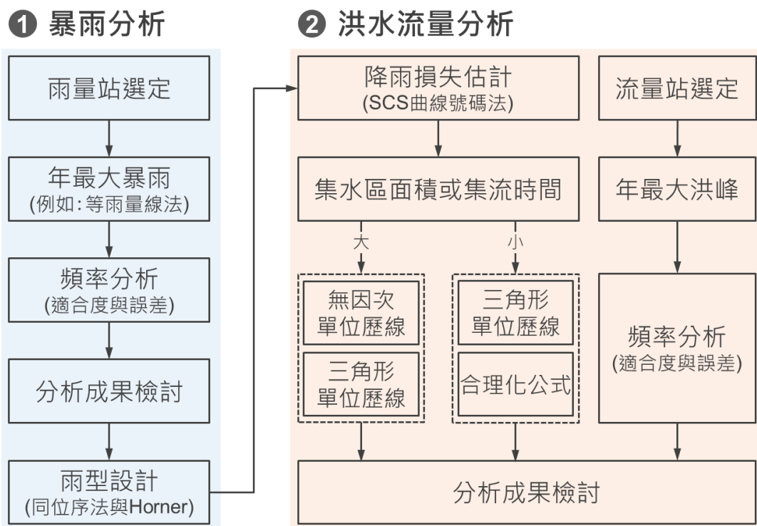
圖 2-1 防洪水文分析架構
