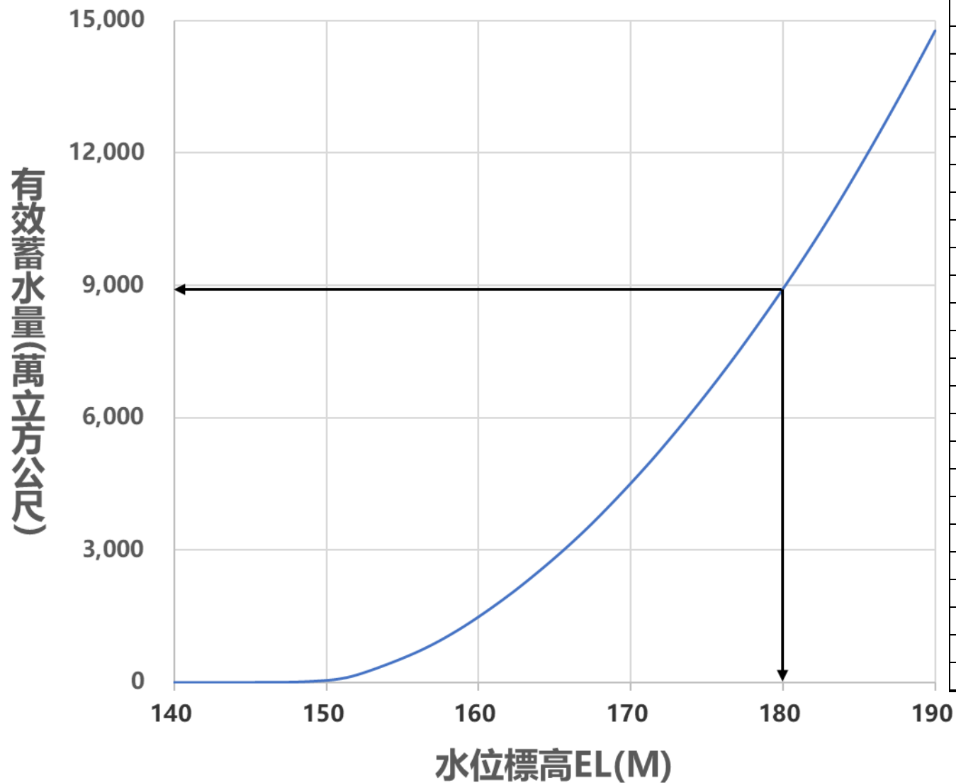
南化水庫水位-蓄水量對照圖
