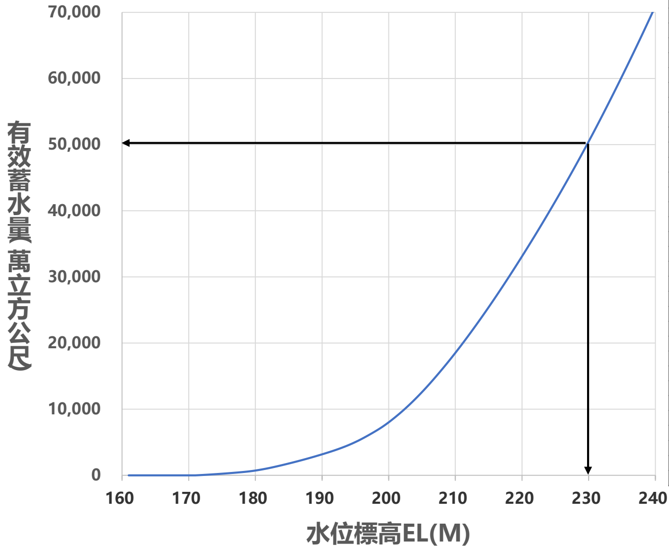
曾文水庫水位-蓄水量對照圖
