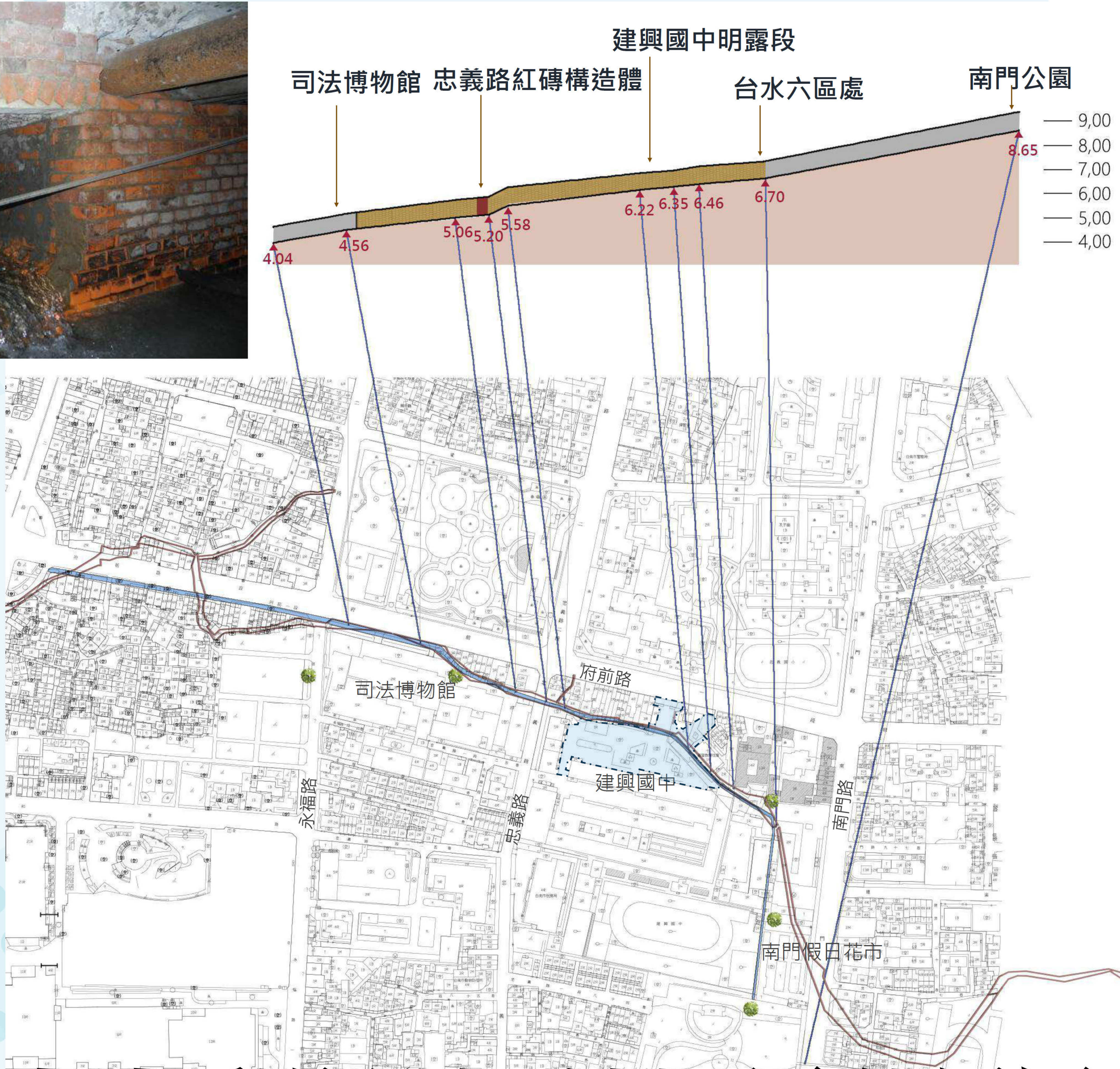
福安坑溪現況水道剖面及位置圖
