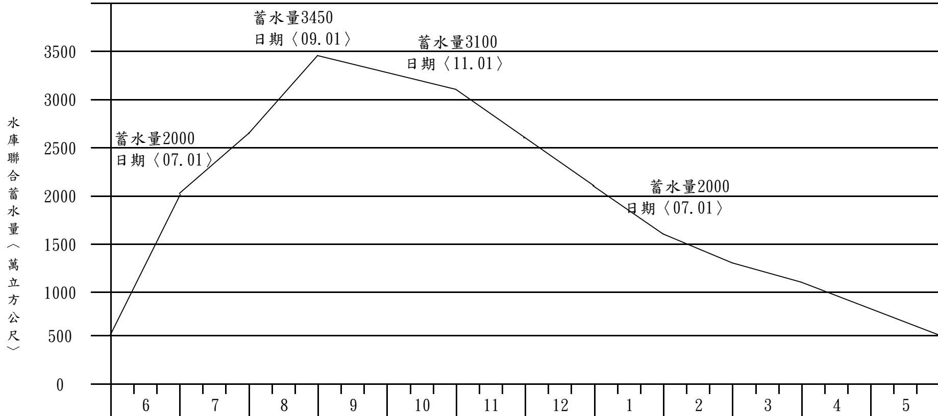
仁義潭、蘭潭水庫串聯聯合運用規線
