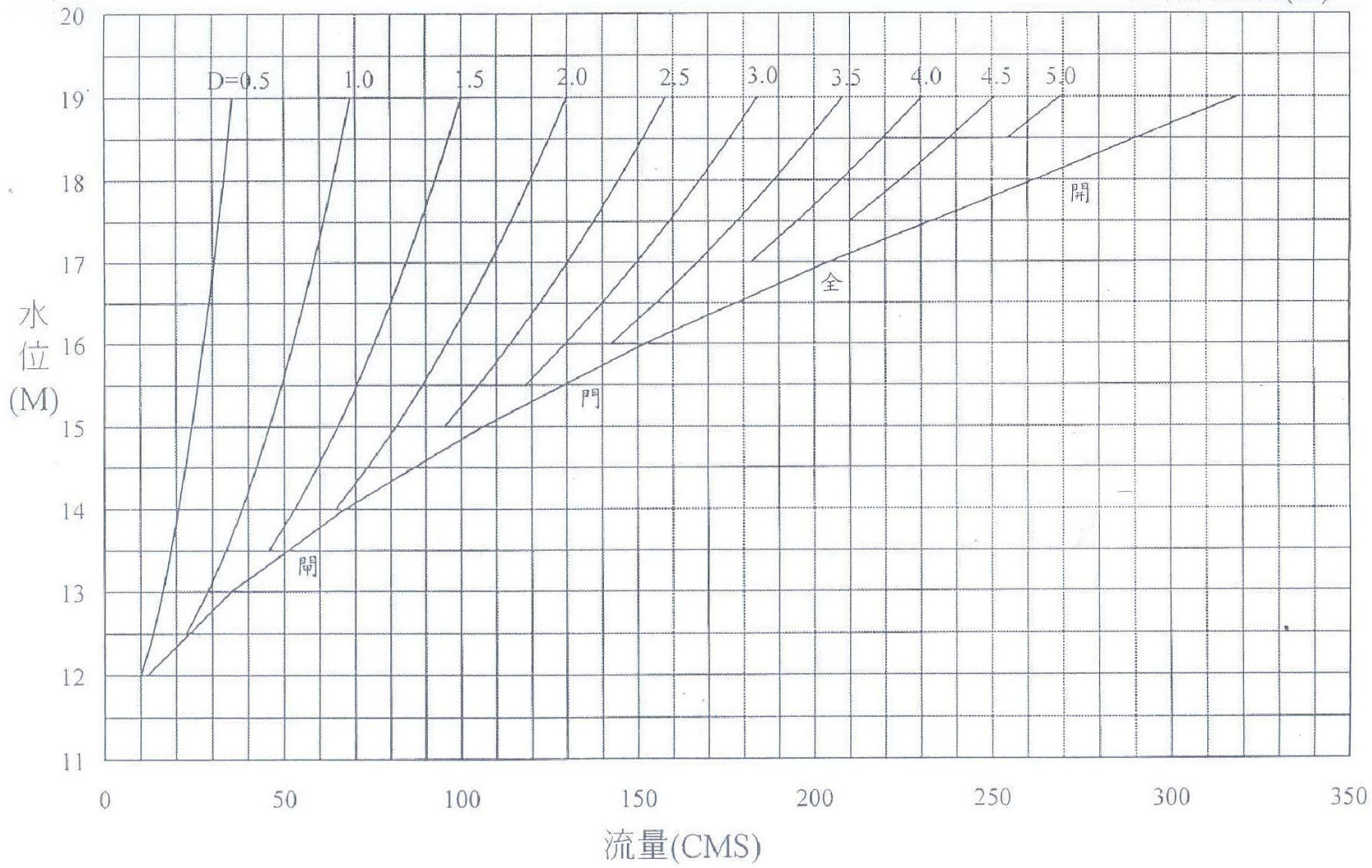
劍潭水庫溢洪道流量率定曲線
