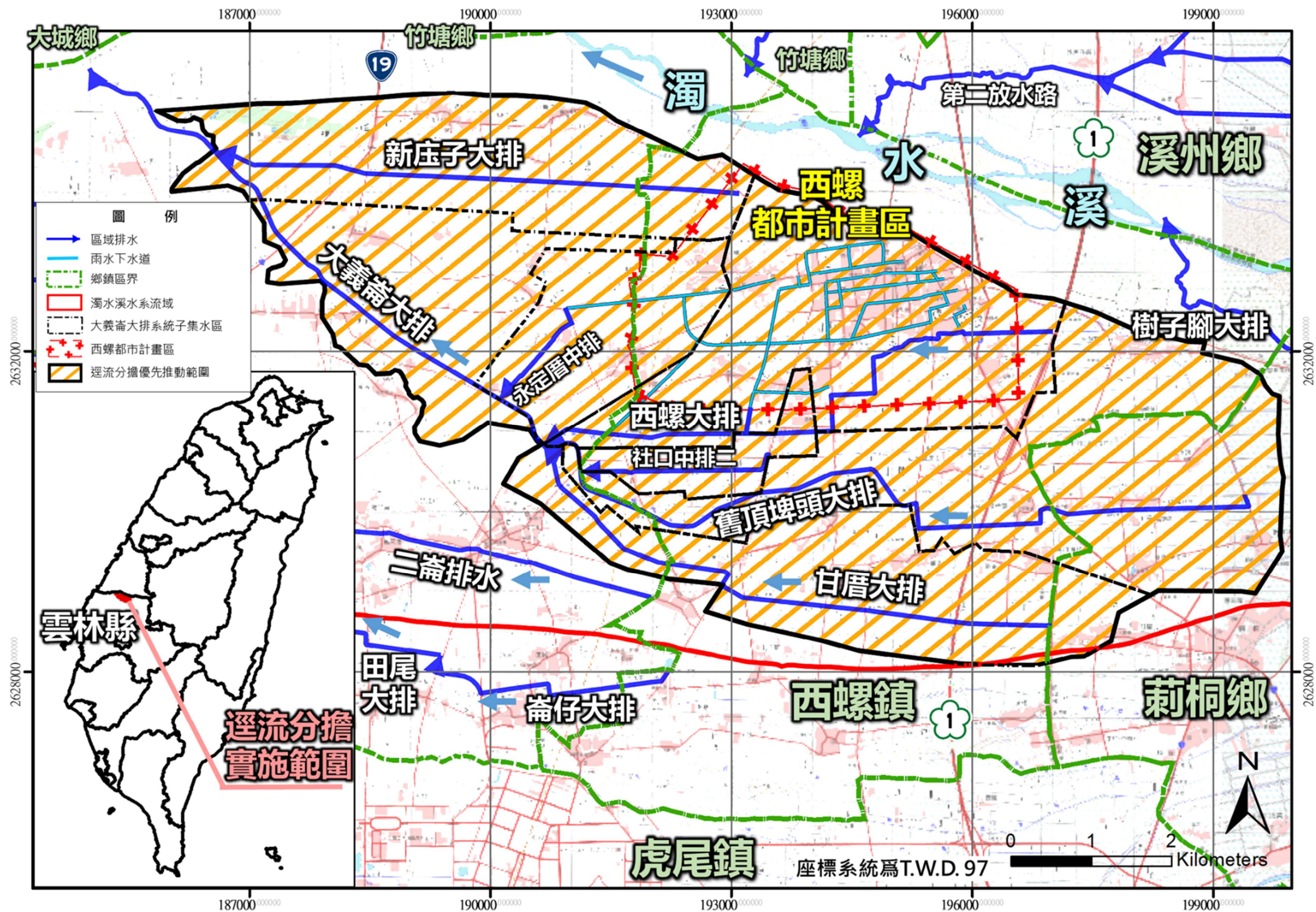
大義崙大排集水區域逕流分擔實施範圍
