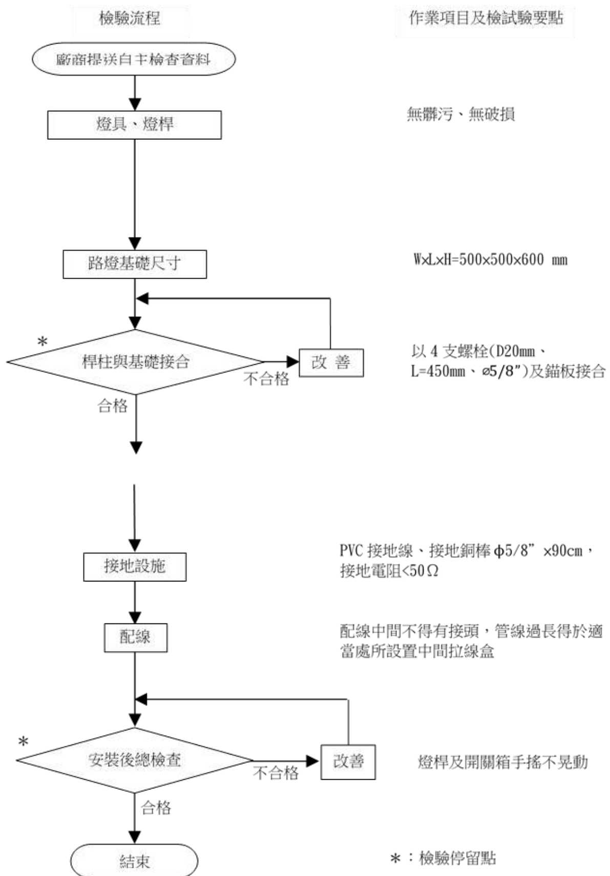
圖 4-9 LED 景觀燈施工檢驗流程圖
