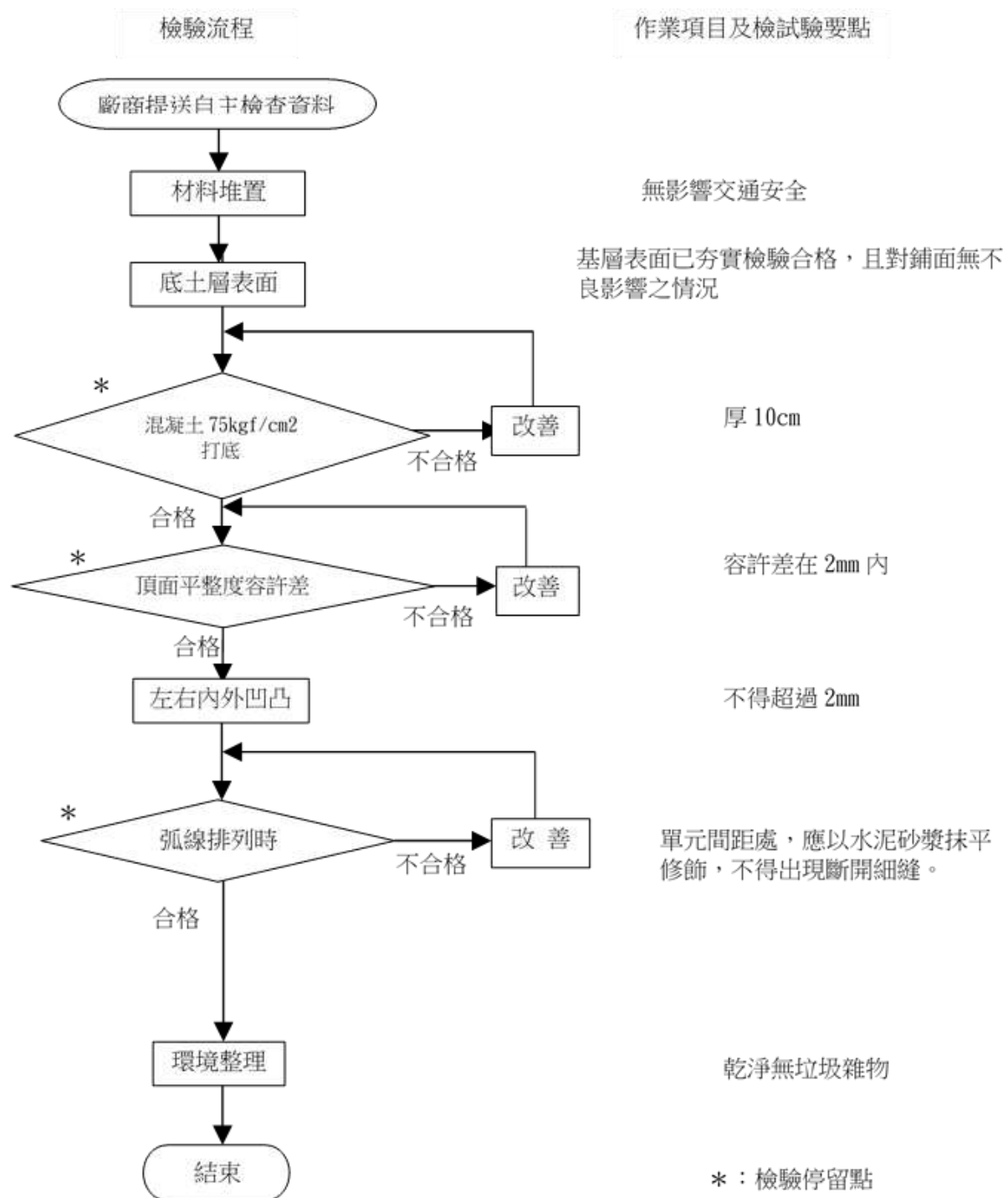
圖 4-13 預鑄路緣石施工檢驗流程圖
