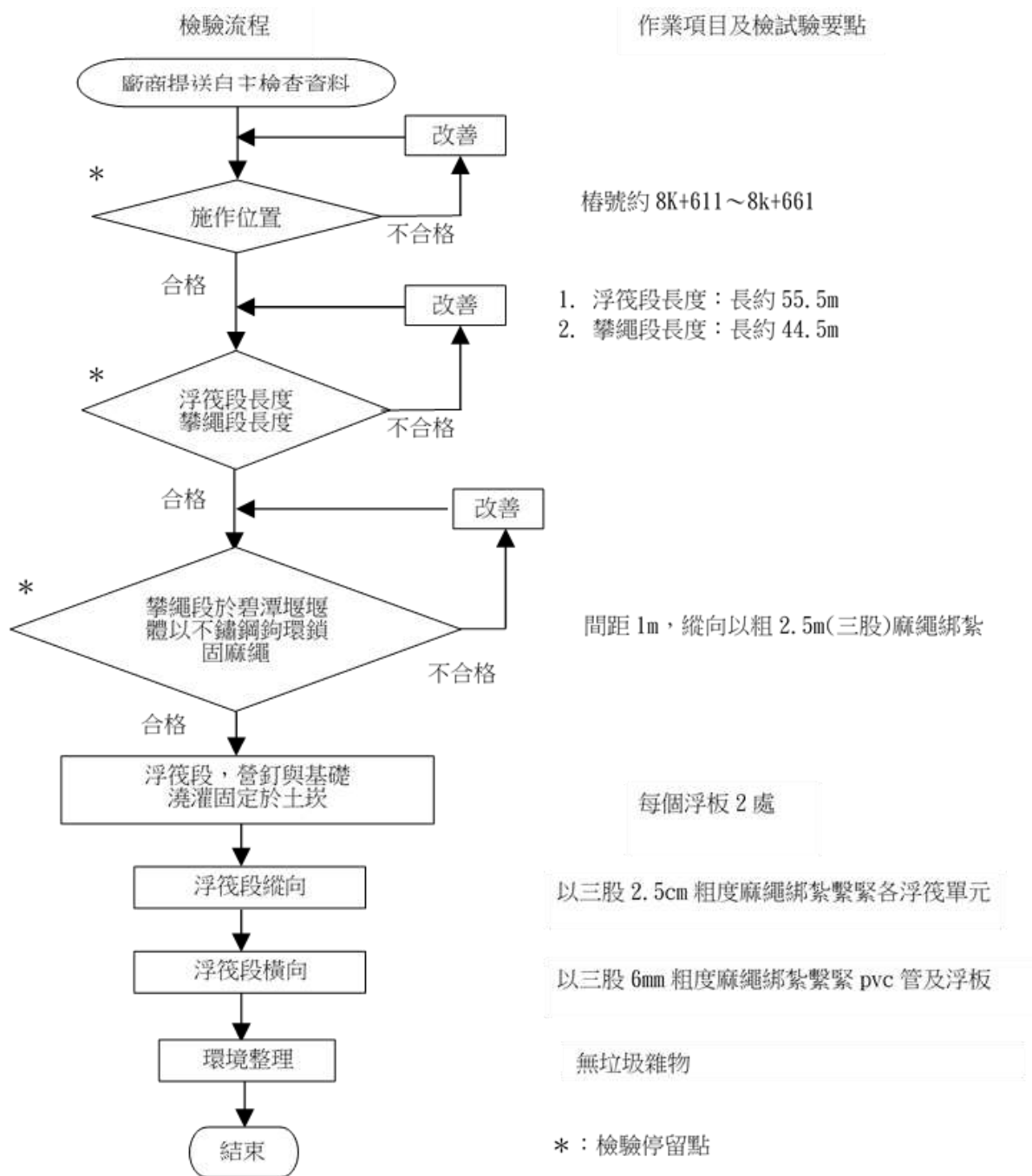
圖 4-20 毛蟹通道施工檢驗流程圖
