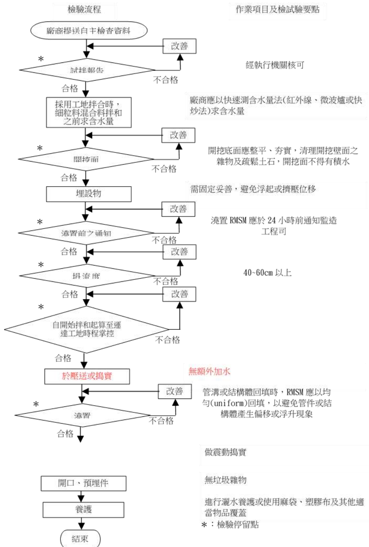
圖 4-5 預拌土壤材料(RSM)施工檢驗流程圖
