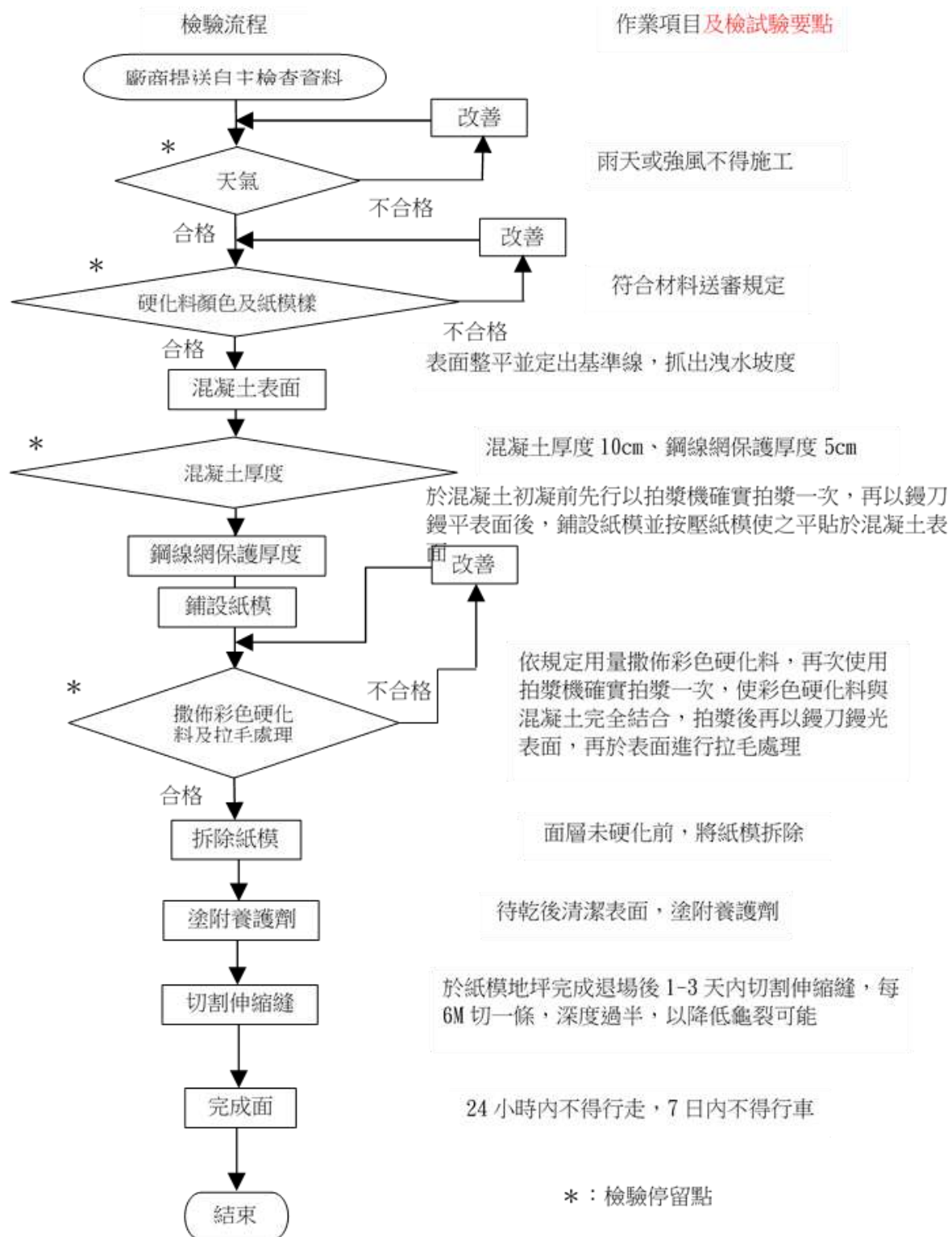
圖 4-11 濕式紙模施工檢驗流程圖
