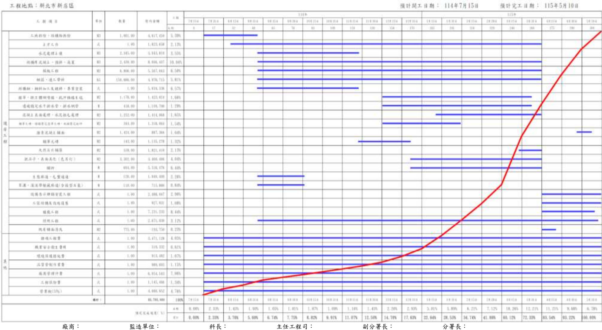
圖 8-1 施工預定進度桿狀圖
