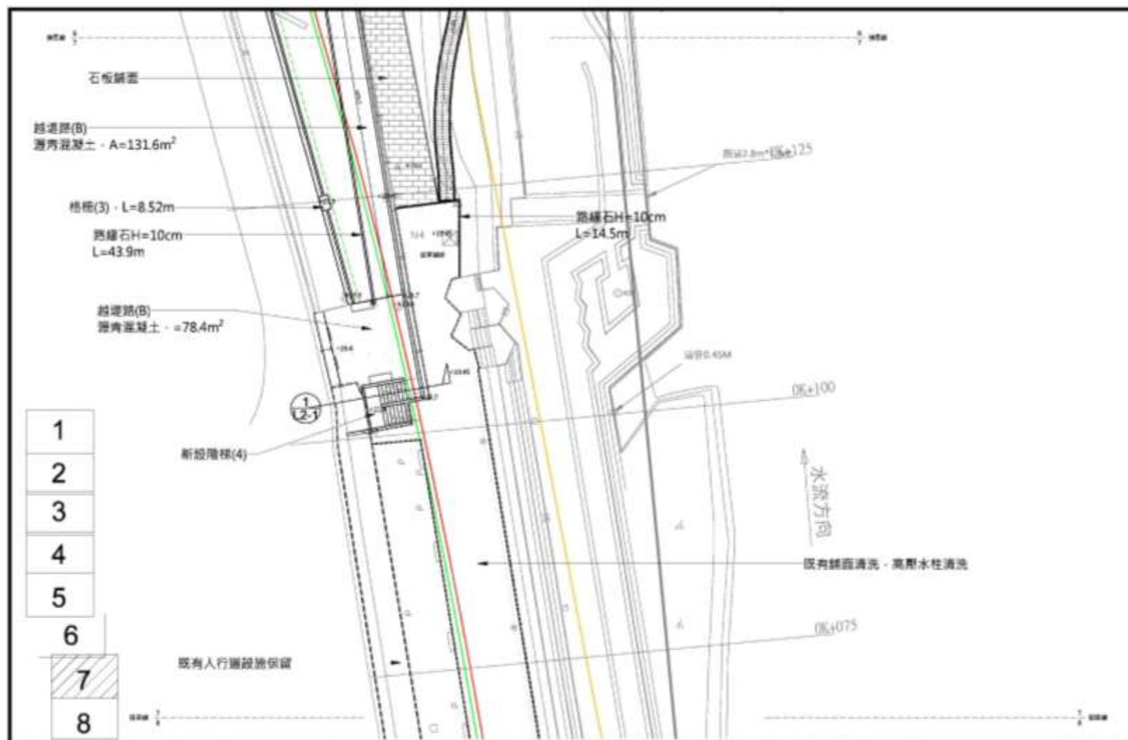
圖 1-1 平面配置圖(7/8)
