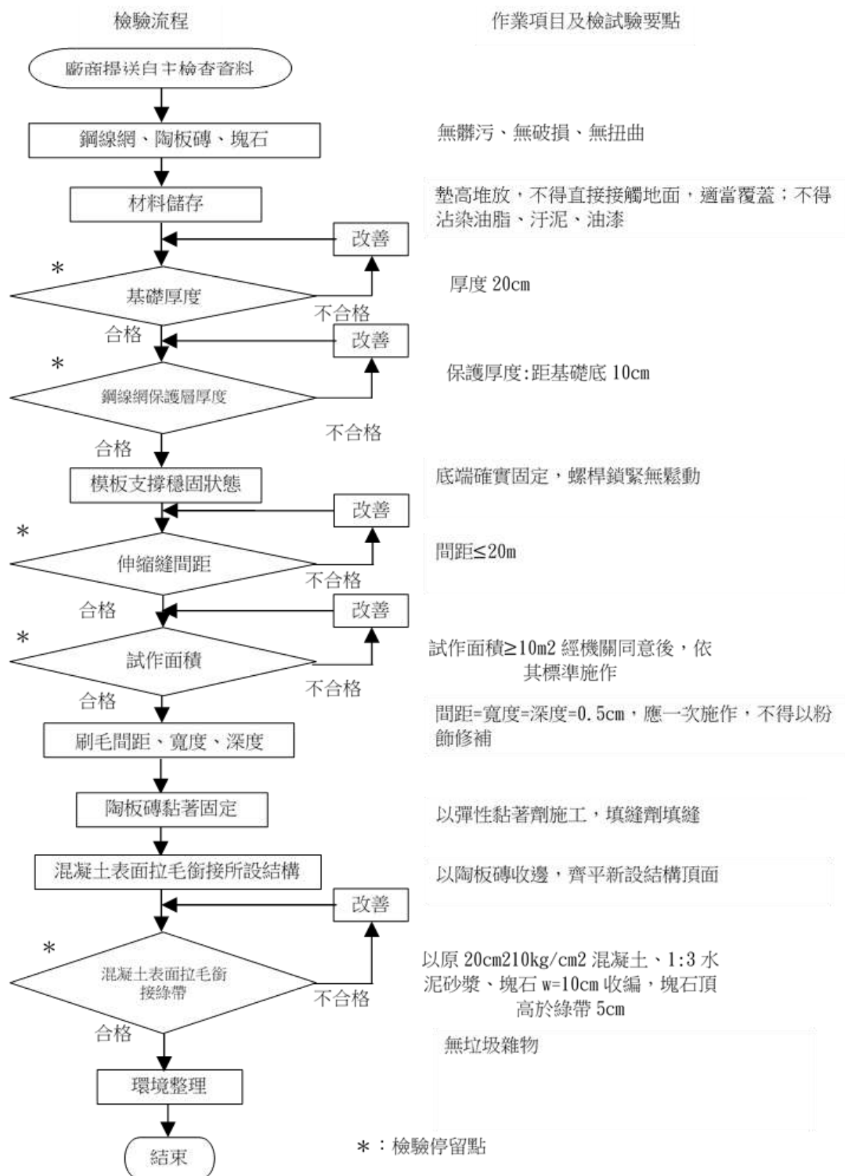
圖 4-19 混凝土拉毛施工檢驗流程圖
