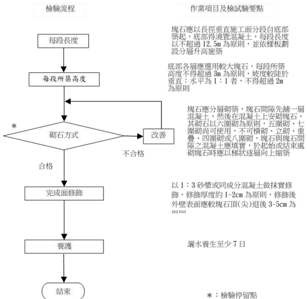
圖 4-16 混凝土砌塊石施工檢驗流程圖(2/2)
