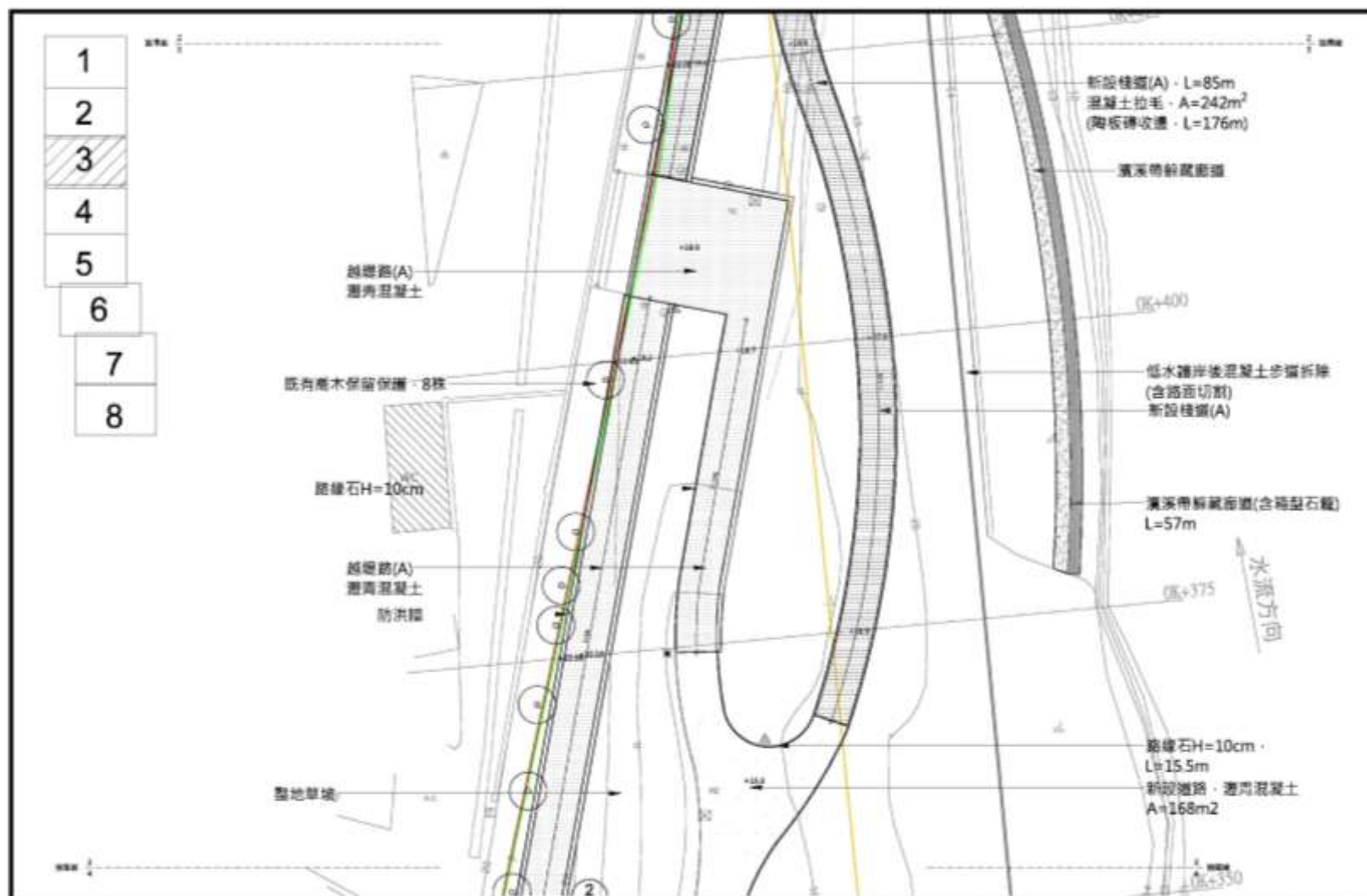
圖 1-1 平面配置圖(3/8)
