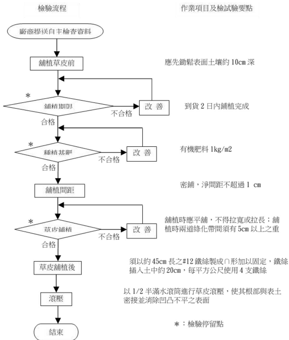
圖 4-8 鋪草皮施工檢驗流程圖
