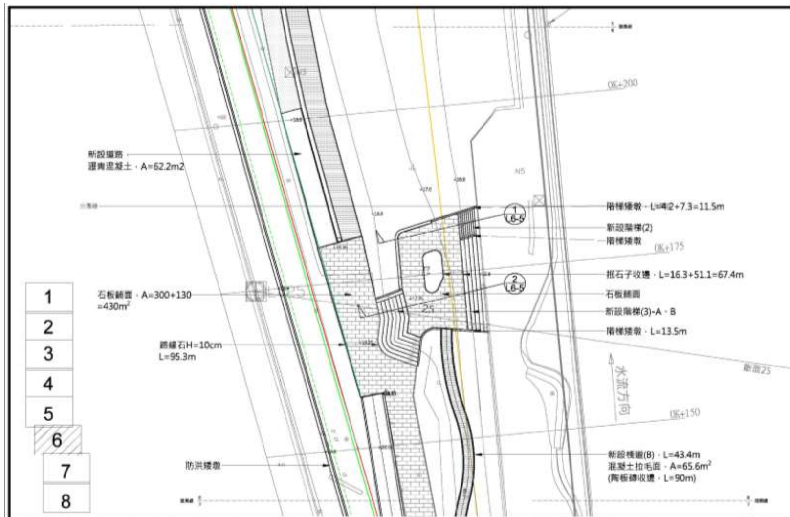
圖 1-1 平面配置圖(6/8)
