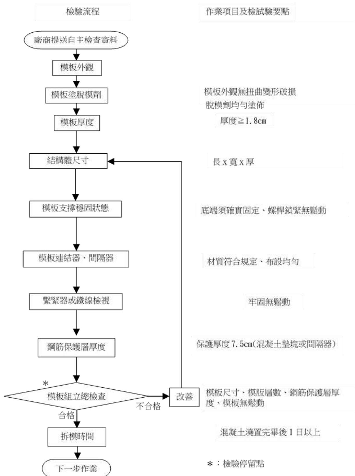
圖 4-23 一般模板施工檢驗流程圖
