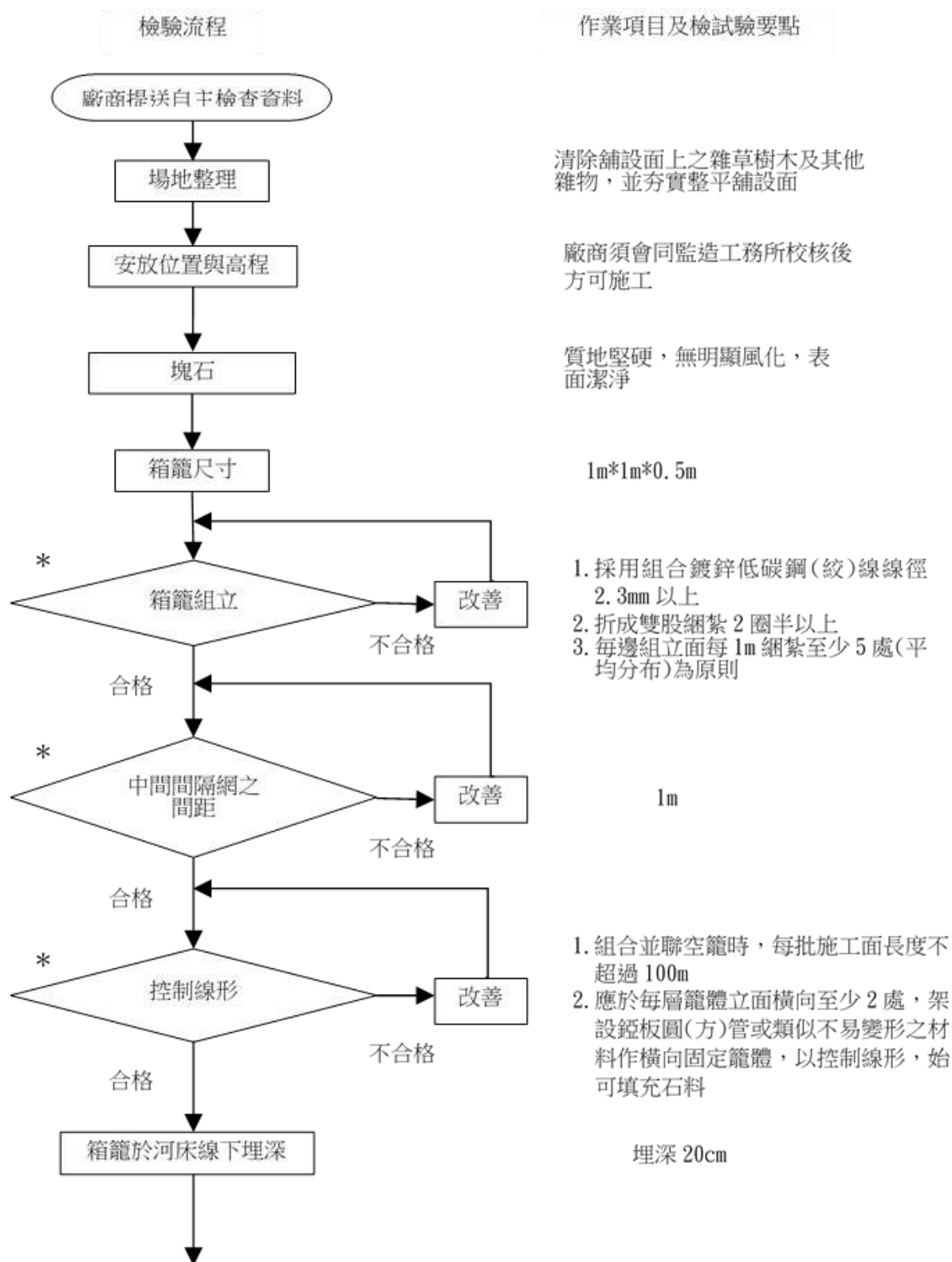
圖 4-17 濱溪帶廊道箱型石籠施工檢驗流程圖(1/2)
