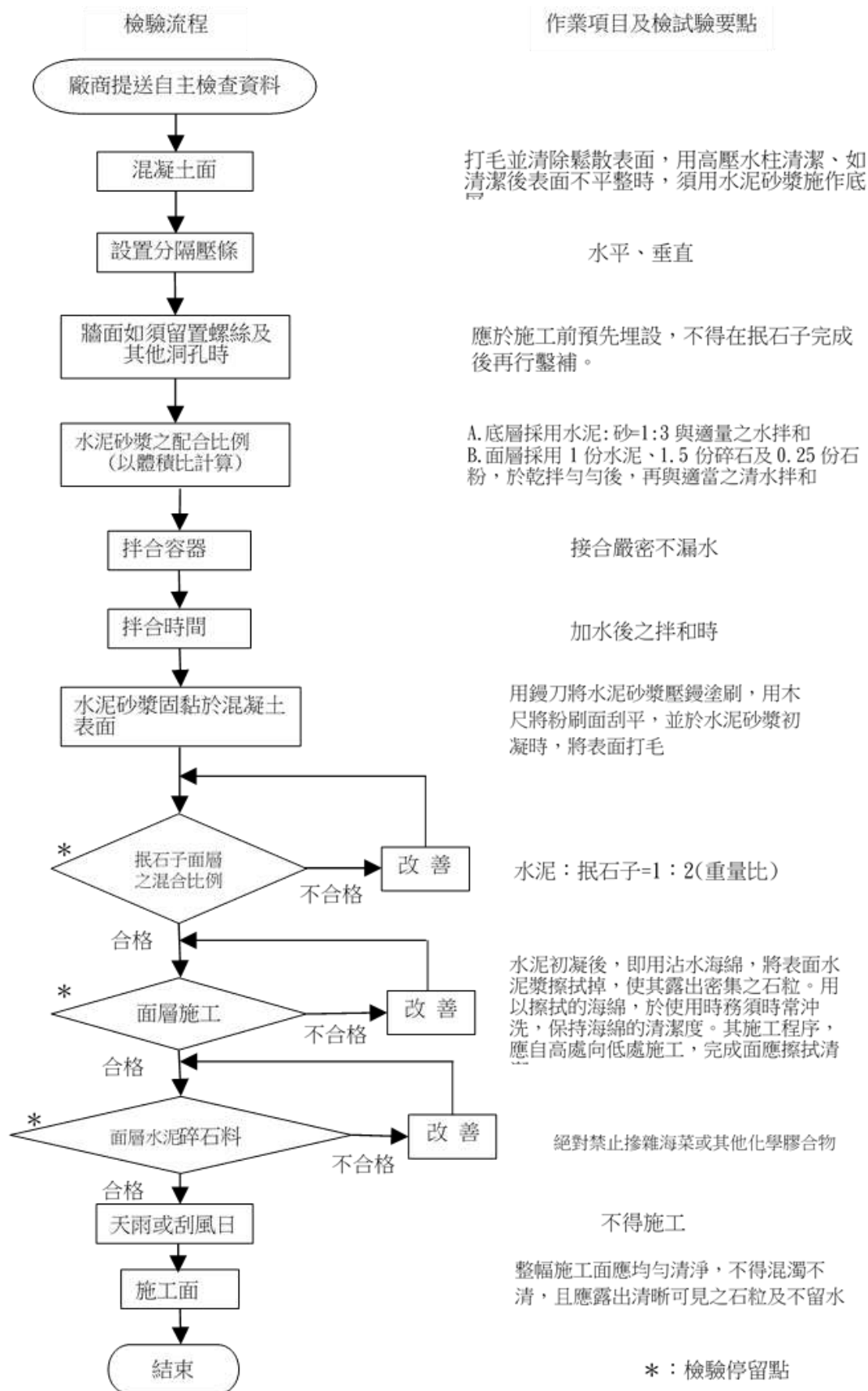
圖 4-15 抵石子施工檢驗流程圖
