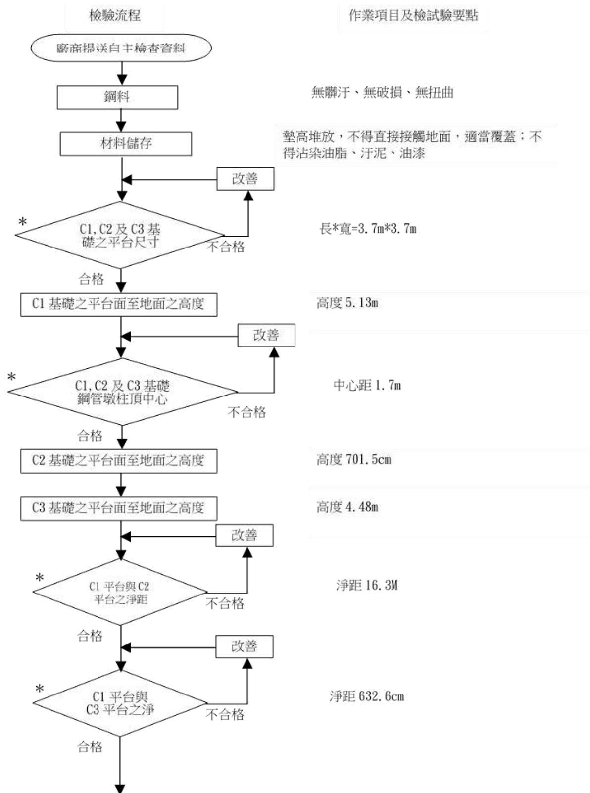
圖 4-24 牽引道(B)立柱及搭接施工檢驗流程圖(1/2)
