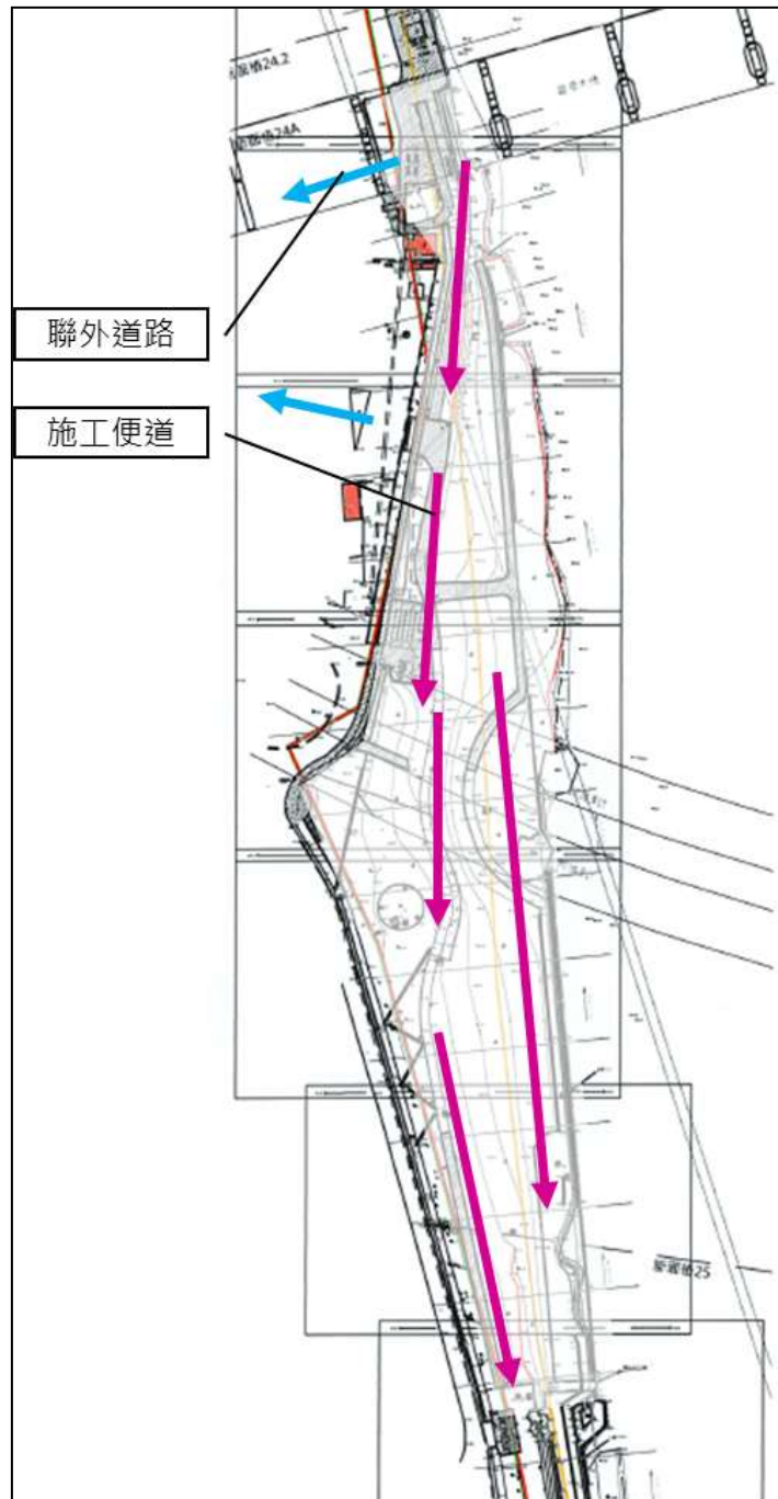
圖 7-1 交通維持計畫圖
