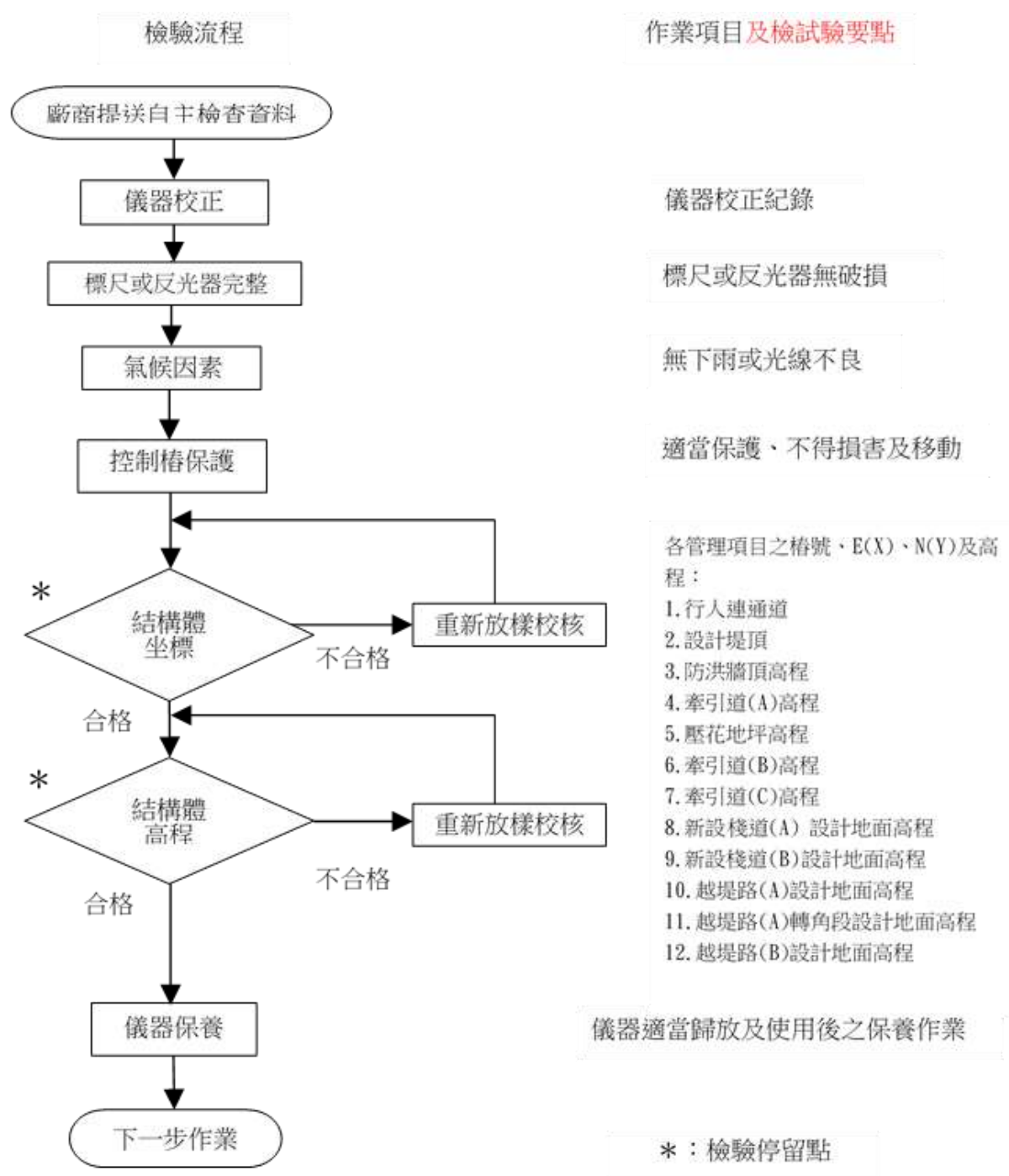
圖 4-2 測量放樣施工檢驗流程圖
