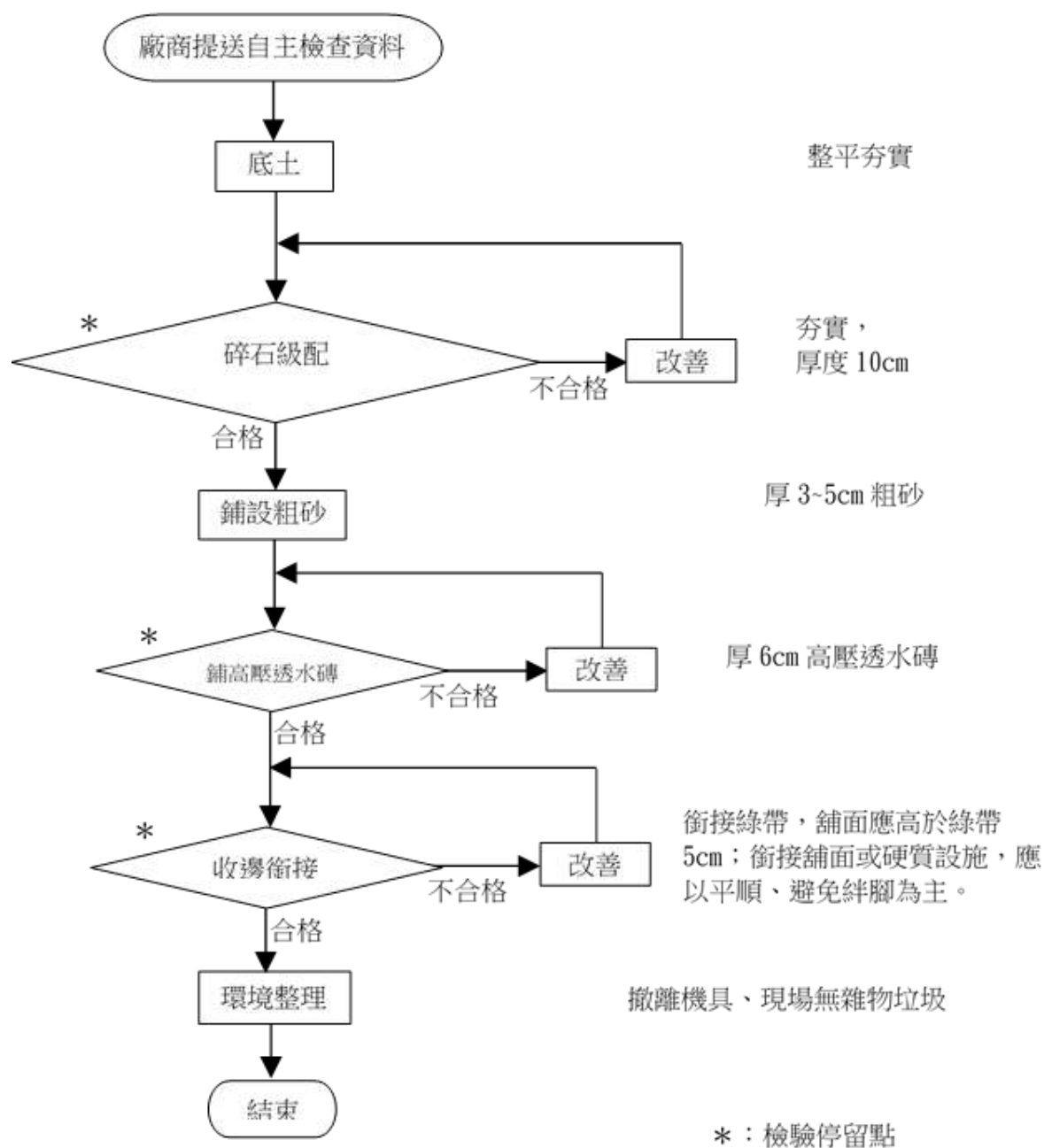
圖 4-12-1 高壓磚及石板鋪面(高壓混凝土磚)施工檢驗流程圖
