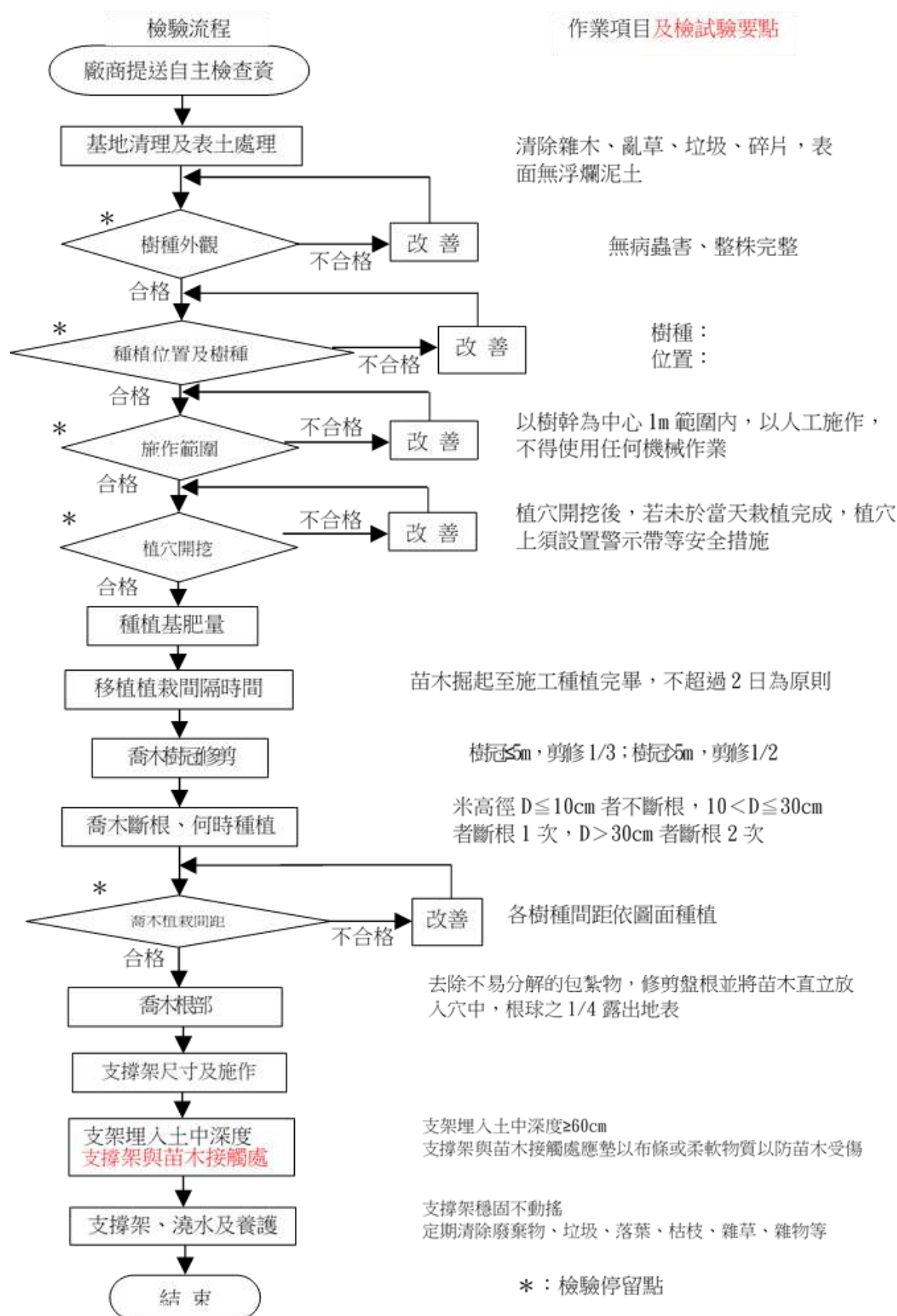
圖 4-6 新植喬木施工檢驗流程圖
