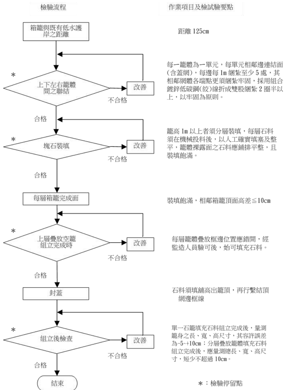
圖 4-17 濱溪帶廊道箱型石籠施工檢驗流程圖(2/2)
