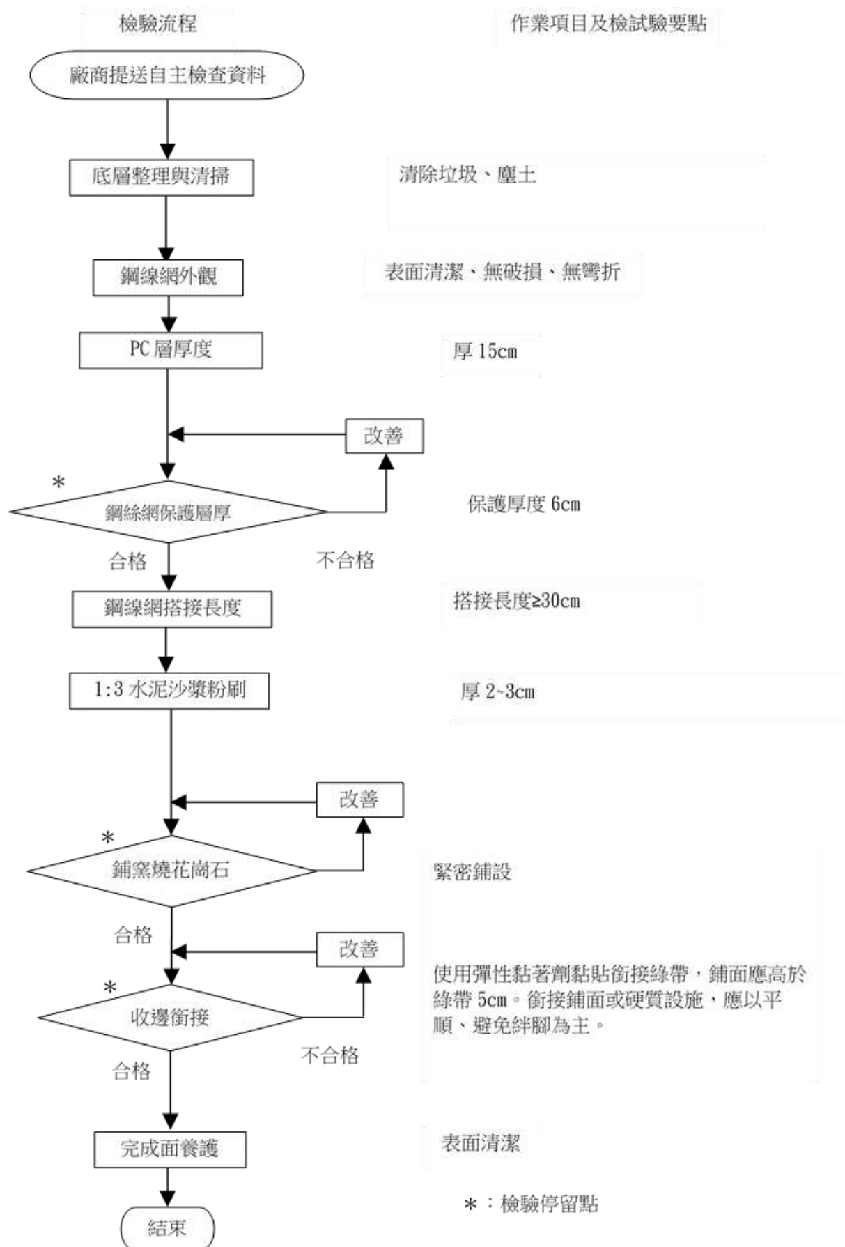
圖 4-12-3 高壓磚及石板鋪面(窯燒花崗石)鋪面施工檢驗流程圖
