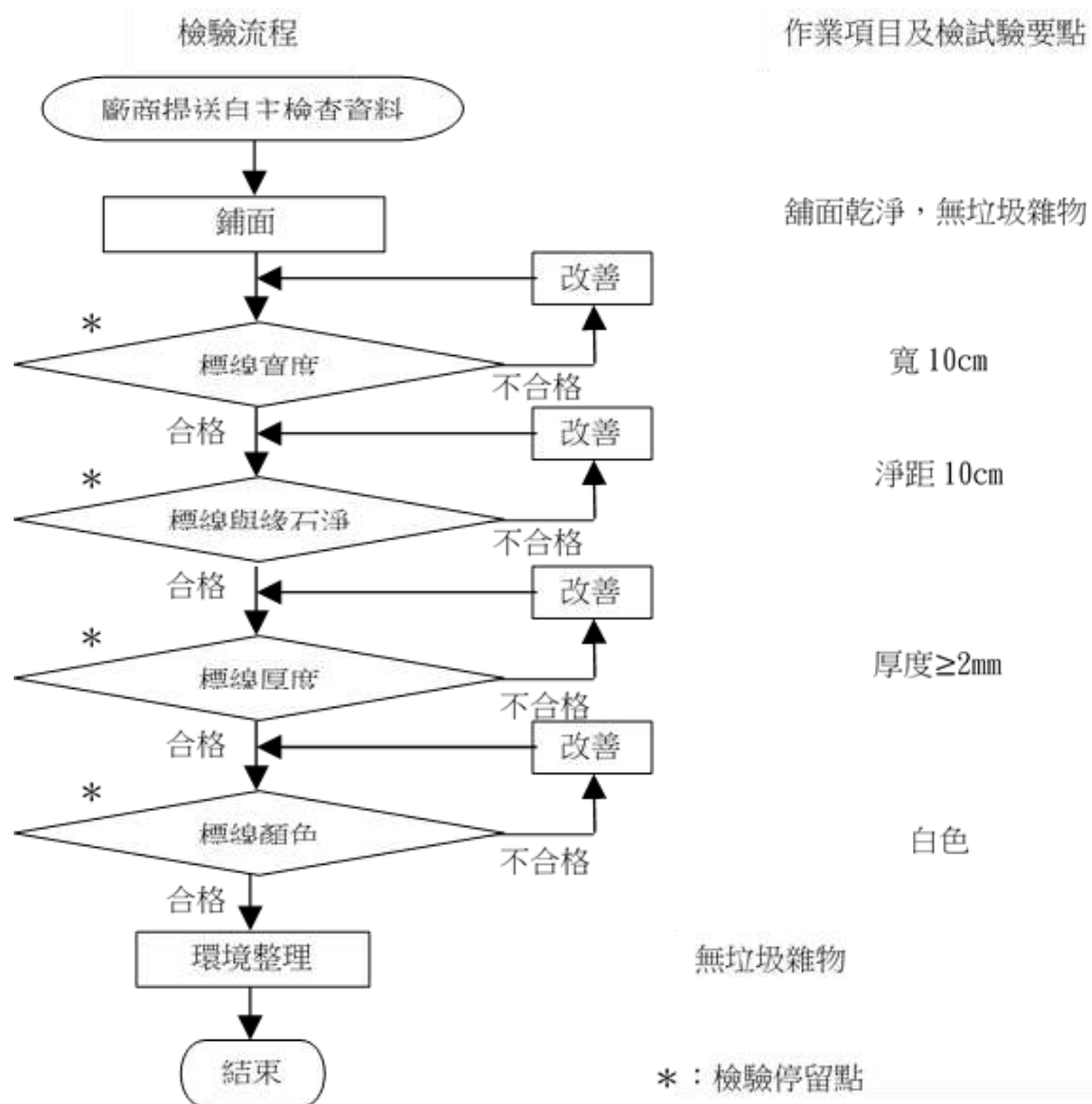
圖 4-18 標線施工檢驗流程圖
