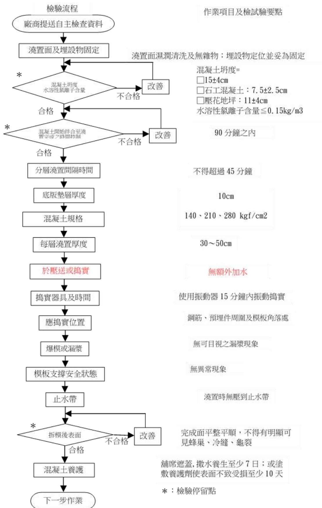
圖 4-21 一般混凝土施工檢驗流程圖
