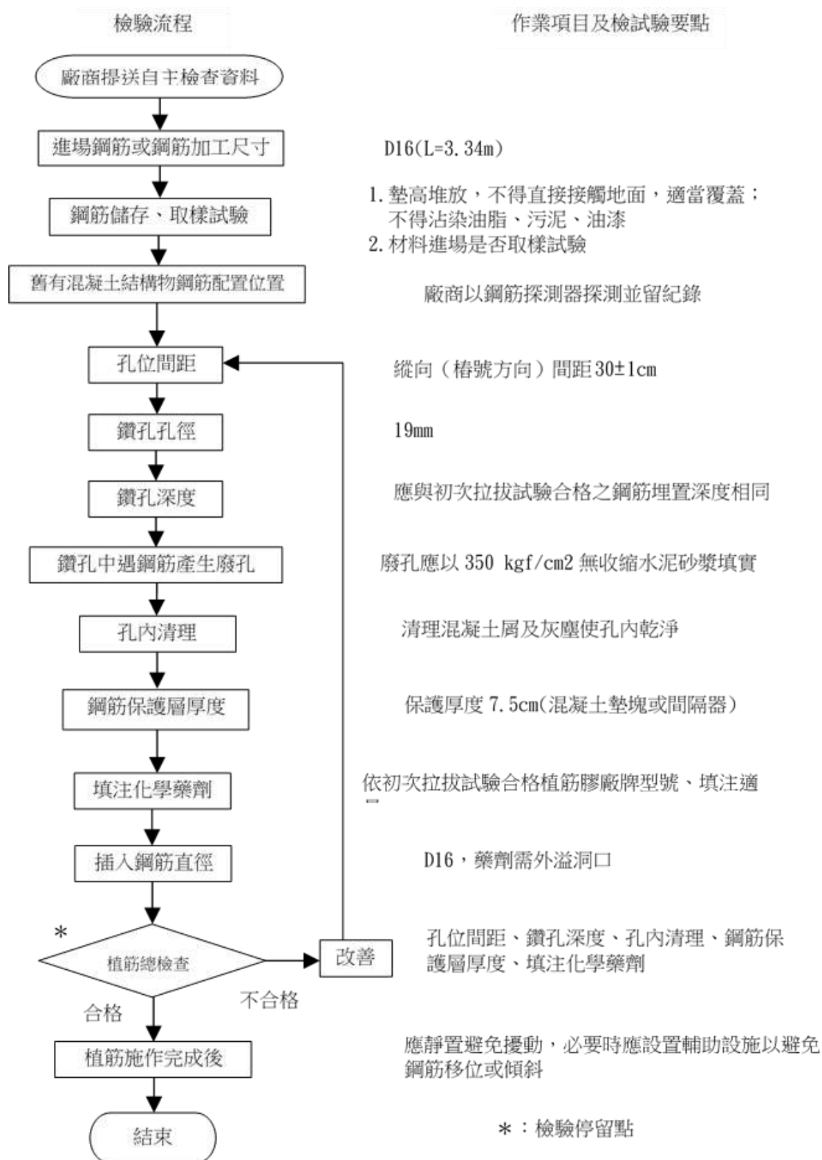
圖 4-25 植筋施工檢驗流程圖
