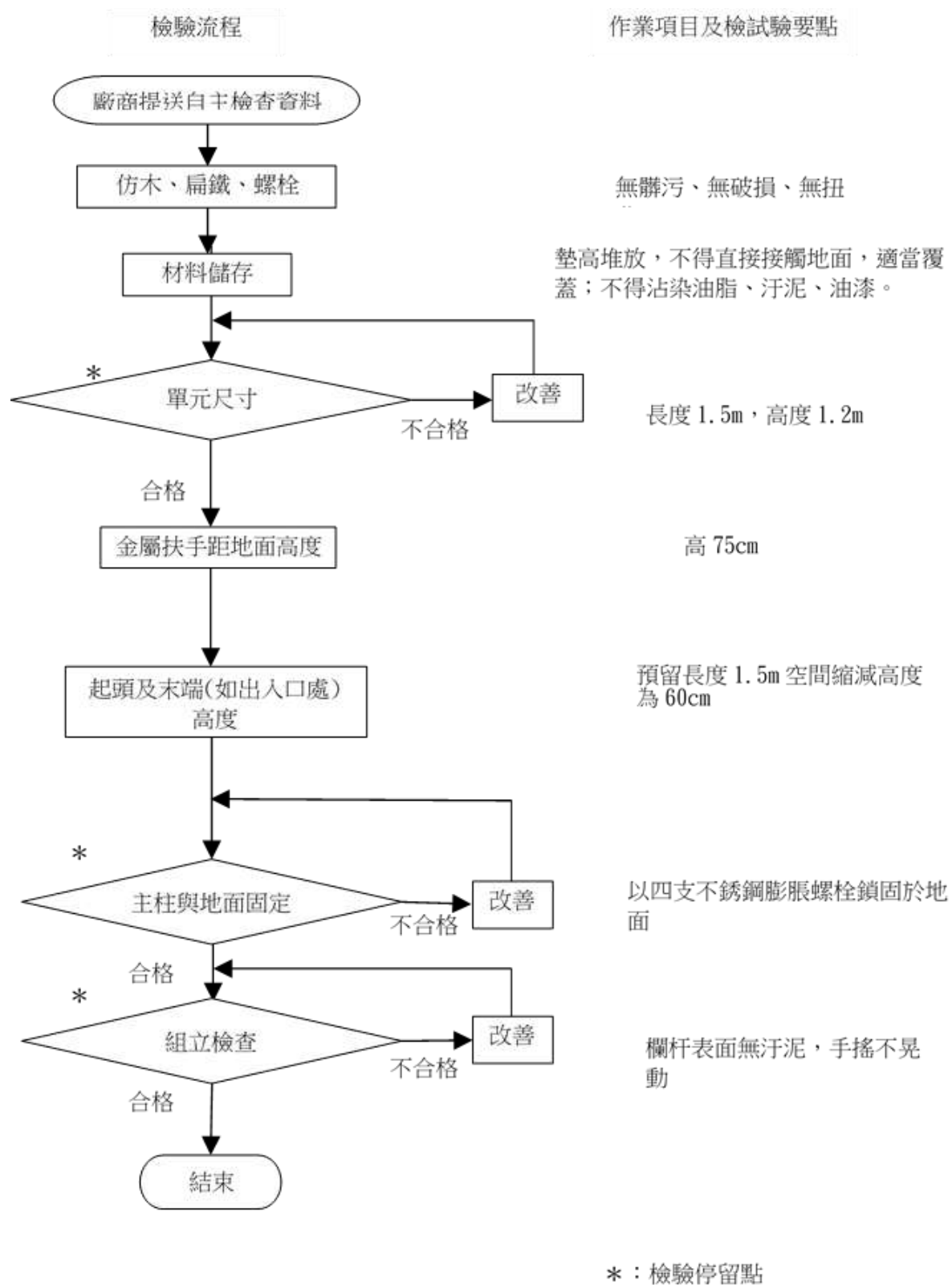
圖 4-14 欄杆施工檢驗流程圖
