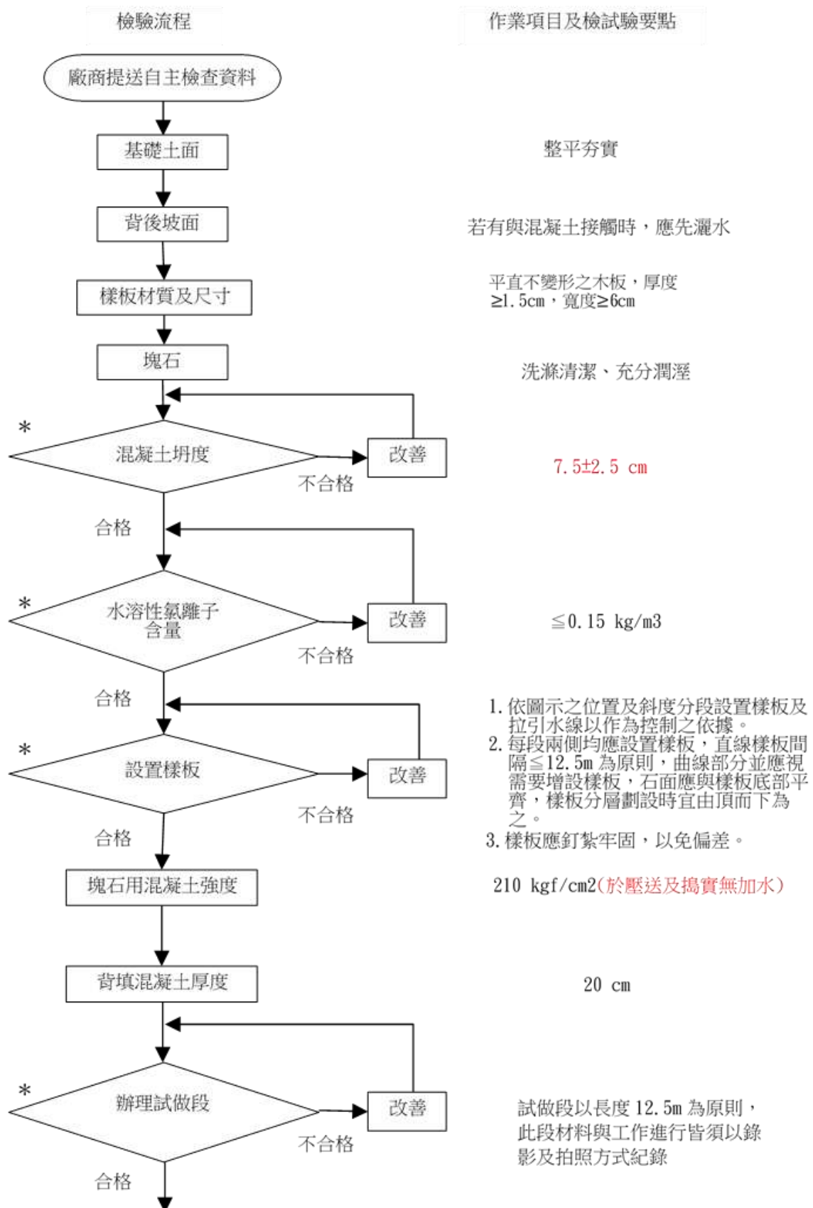
圖 4-16 混凝土砌塊石施工檢驗流程圖(1/2)
