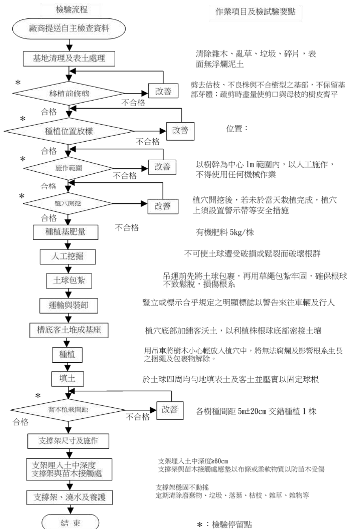
圖 4-7 移植喬木施工檢驗流程圖
