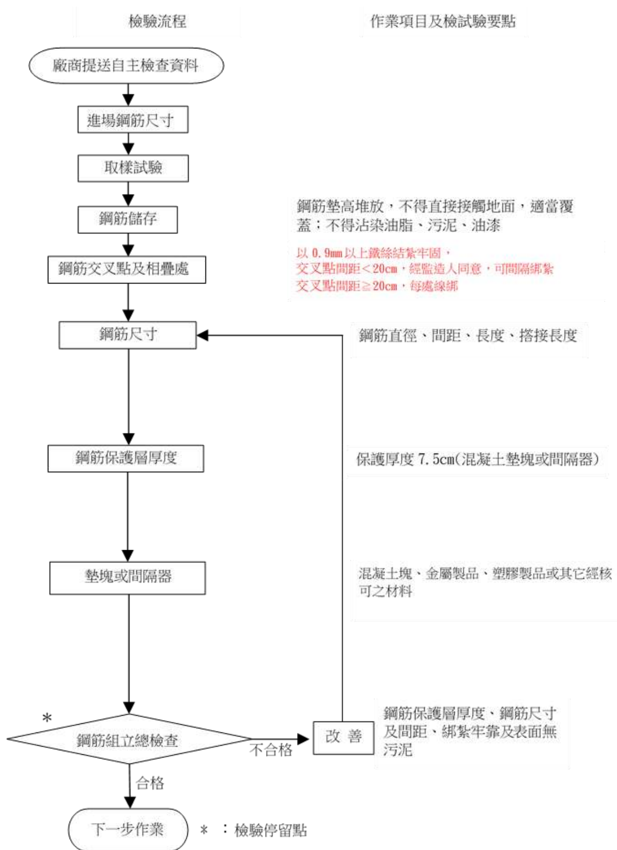
圖 4-22 一般鋼筋施工檢驗流程圖
