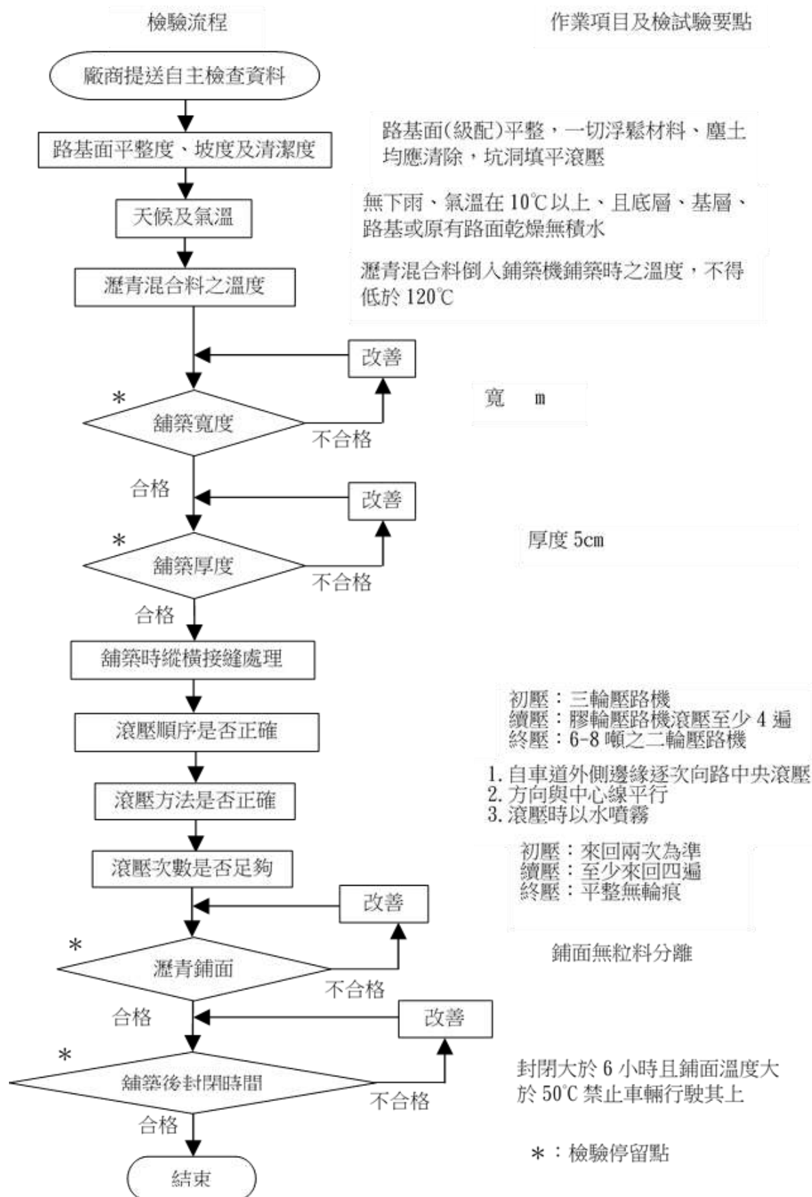
圖 4-10 瀝青混凝土鋪面施工檢驗流程圖
