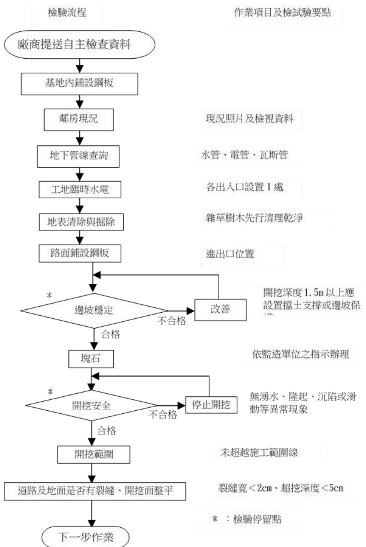
圖 4-3 挖方施工檢驗流程圖
