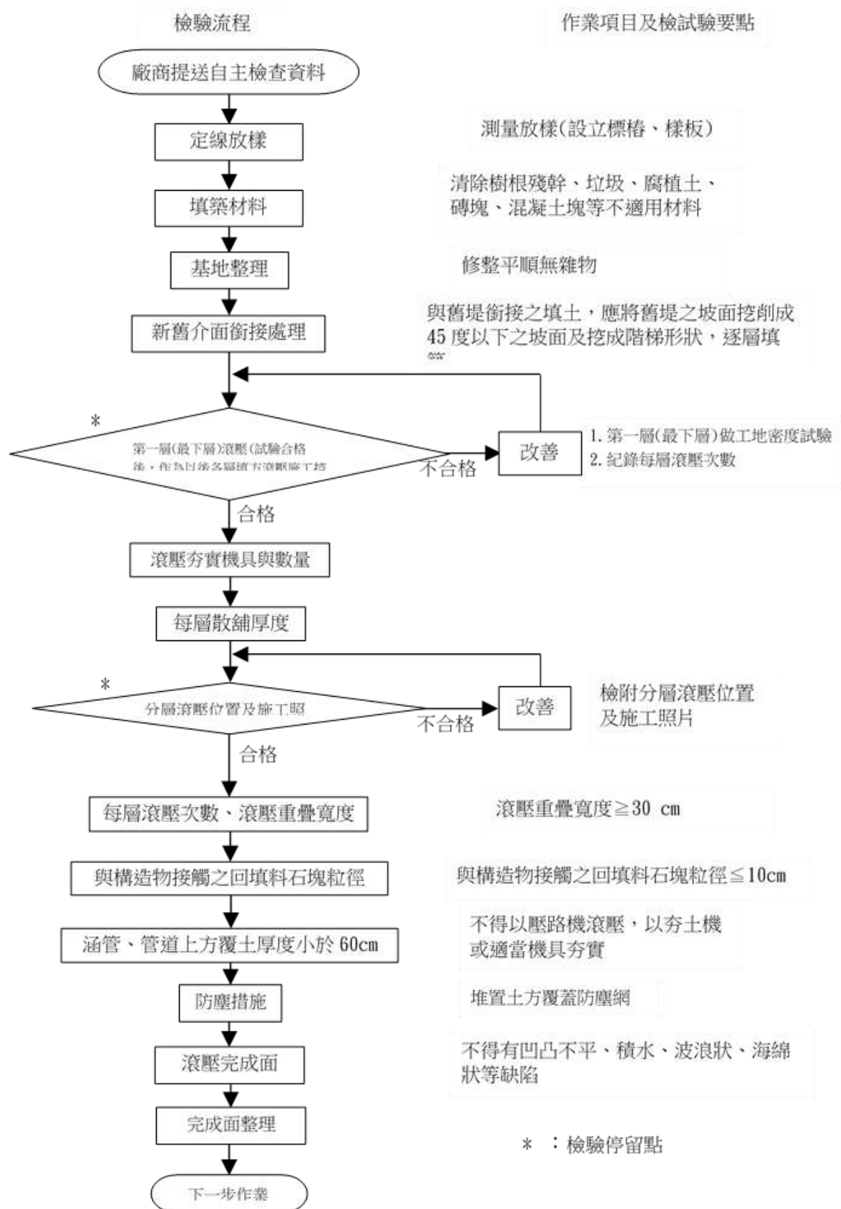
圖 4-4 填方施工檢驗流程圖
