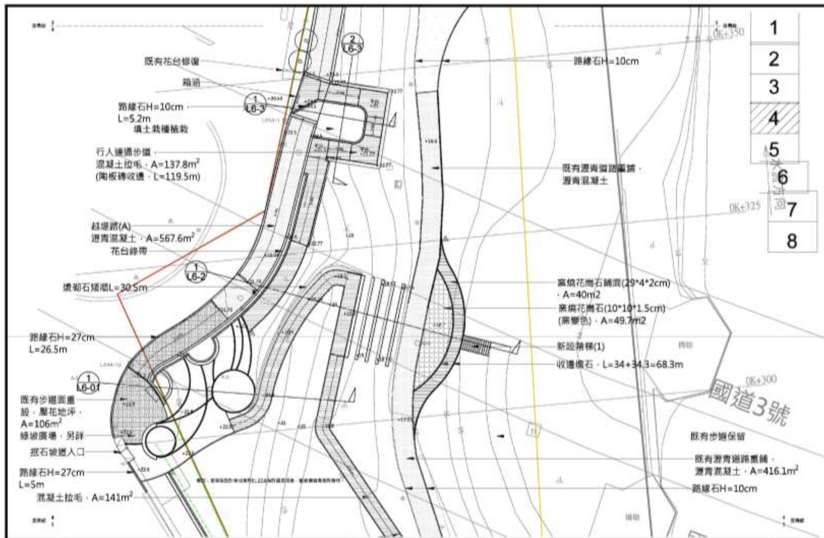
圖 1-1 平面配置圖(4/8)
