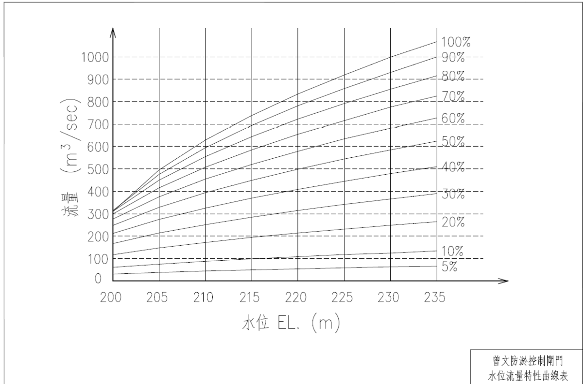
附圖二 防淤隧道閘門開度與流量關係曲線(圖型修正至標高 235 公尺)
