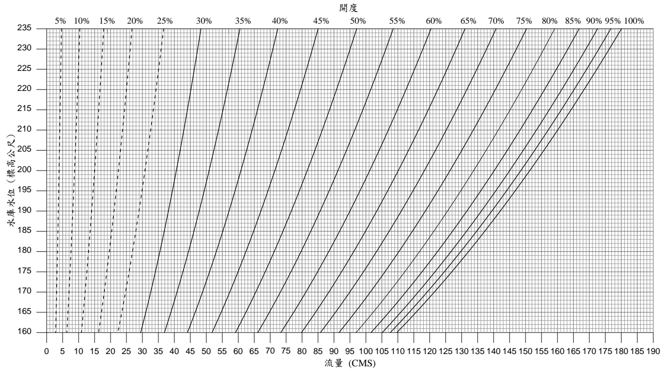
附圖四 射流閘門開度與流量關係曲線(雙閘同時啟閉)
