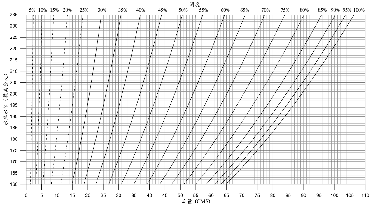
附圖三 射流閘門開度與流量關係曲線(單開啟閉)(圖型修正至標高 235 公尺)
