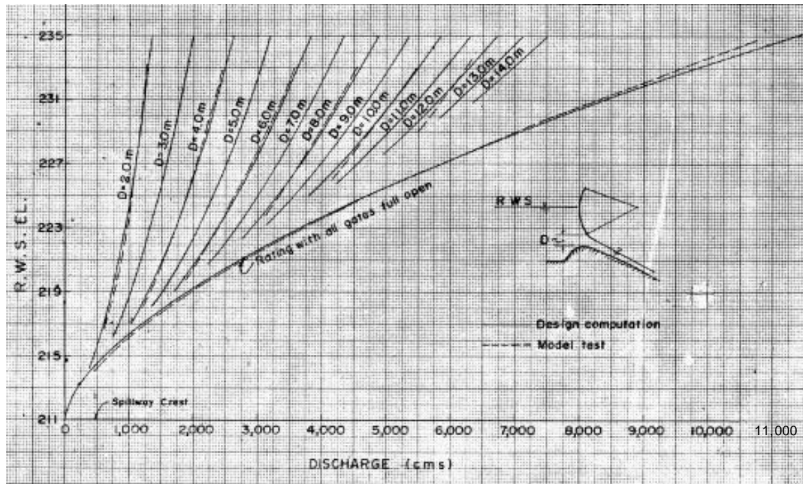
附圖一 溢洪道閘門開度與流量關係曲線(圖型修正至標高 235 公尺)
