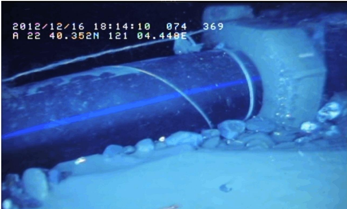
圖附件二-3 水深-369m 處的管線下緣受到沉積物部份填塞
