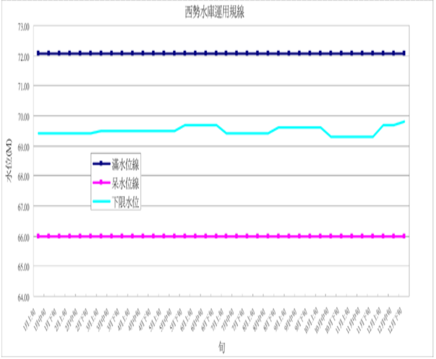
西勢水庫運用規線圖
