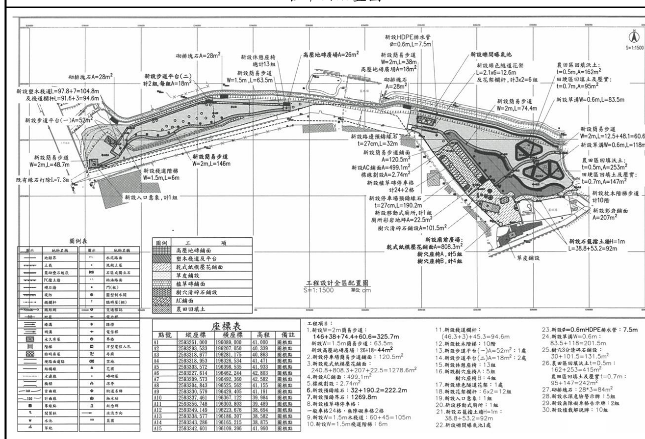
工程平面配置圖
