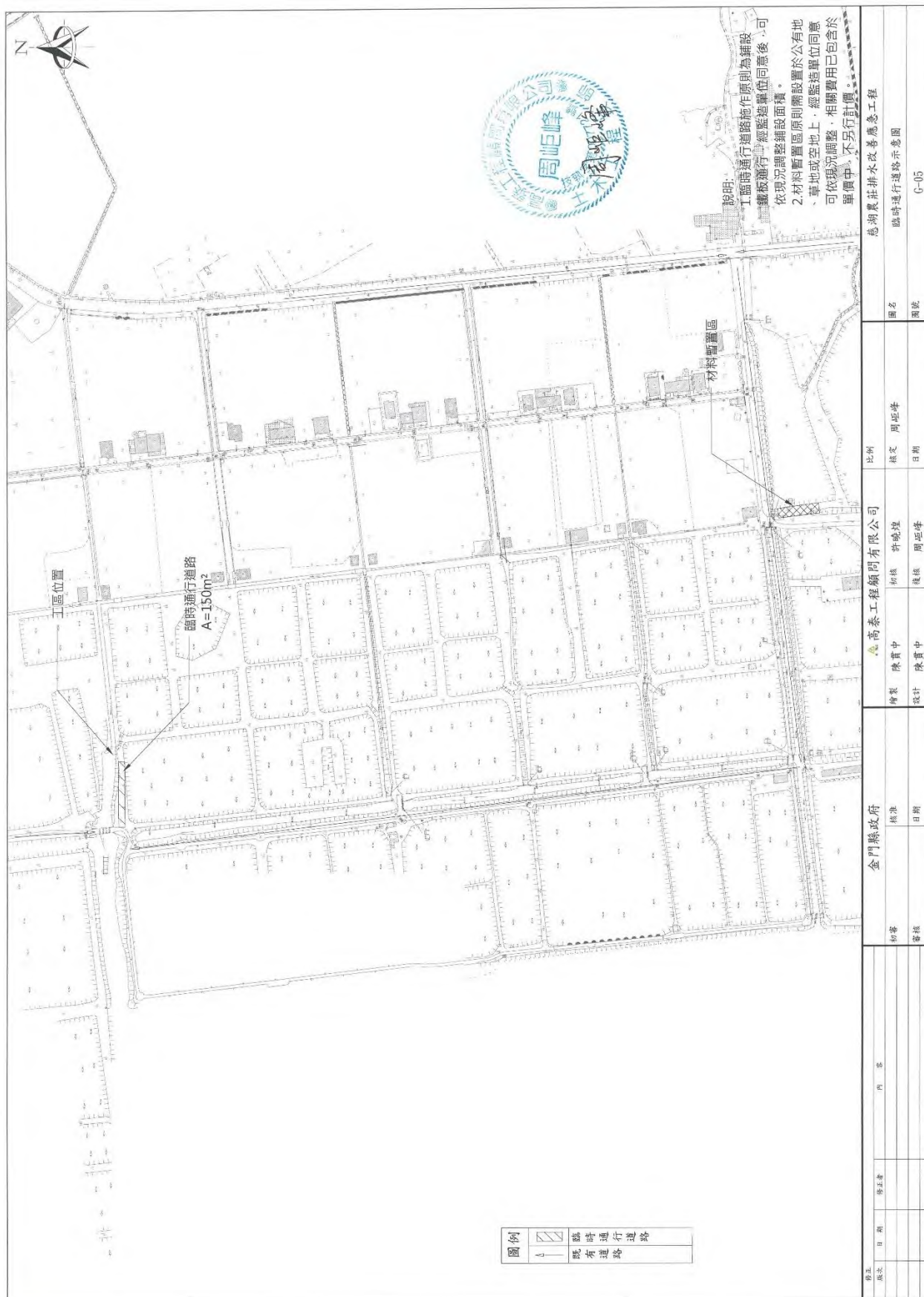
圖 3-47 慈湖農莊排水改善應急工程_施工便道及機具與材料堆置位置平面圖
