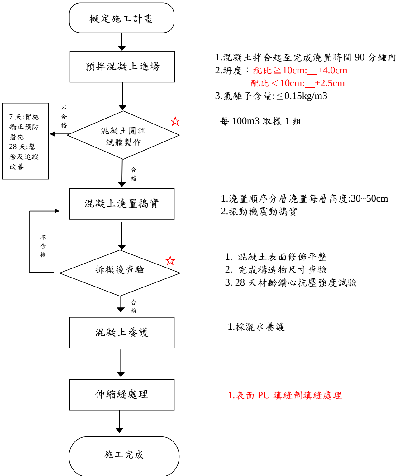
圖三.2 混凝土工程施工檢驗流程
