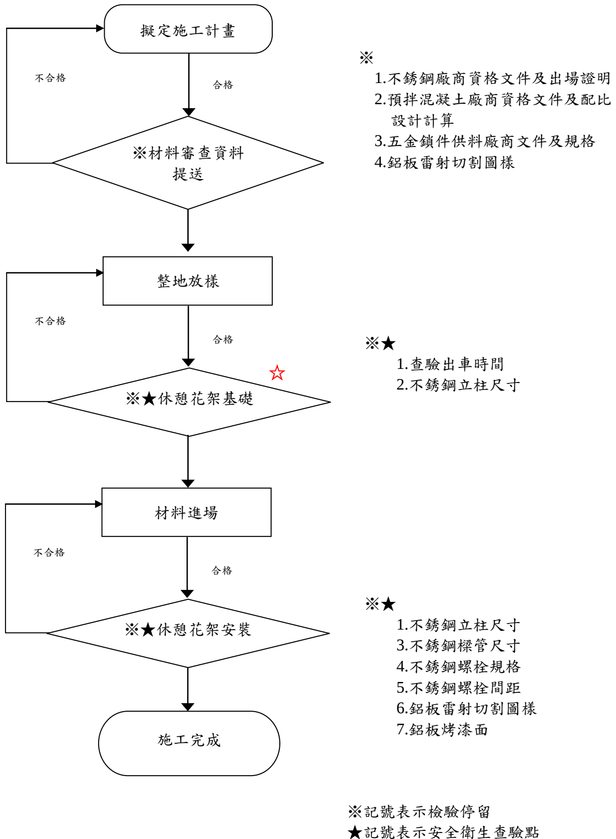
圖 5-12 休憩花架施工檢驗程序
