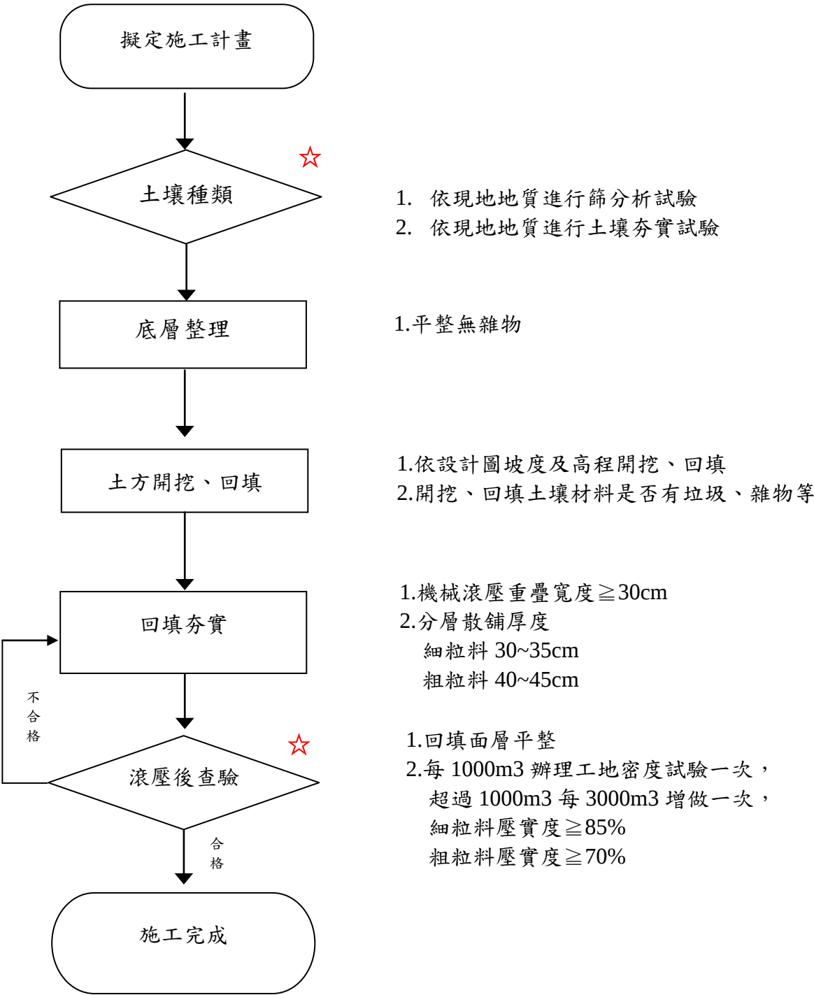
圖三.1 放樣工程施工檢驗流程
