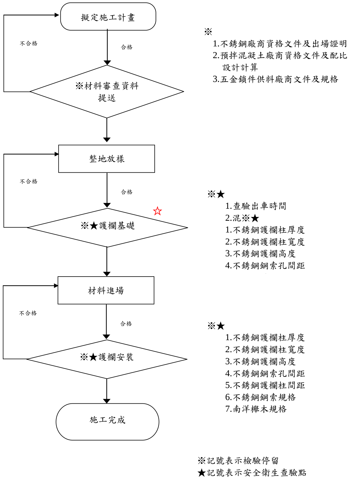
圖 5-11 護欄施工檢驗程序
