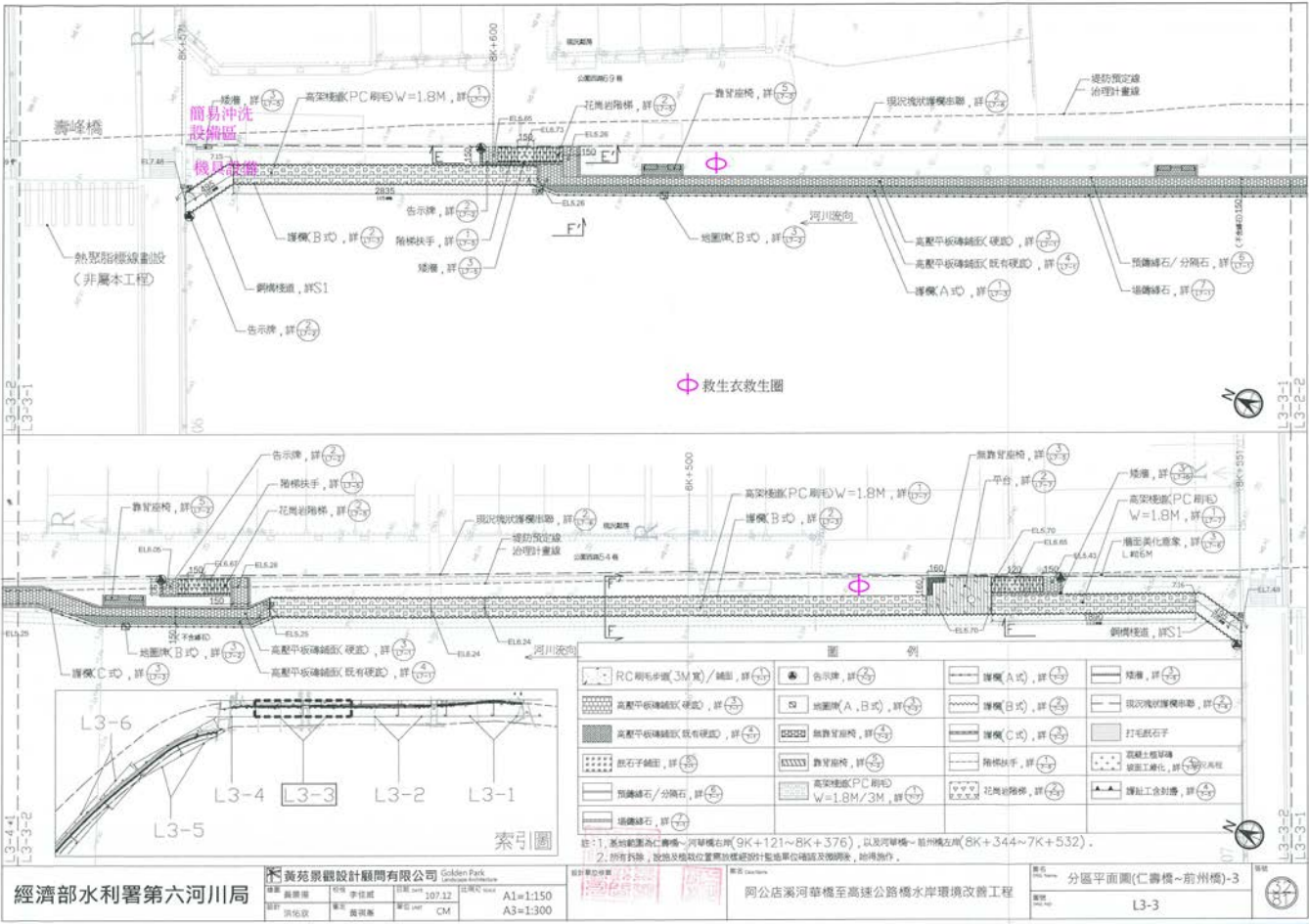
工區規劃布置圖
