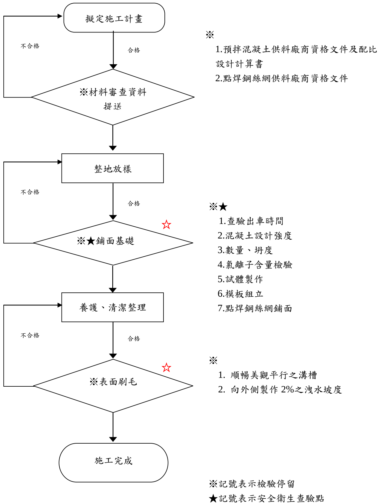
圖三.5 RC 刷毛步道工程施工檢驗程序
