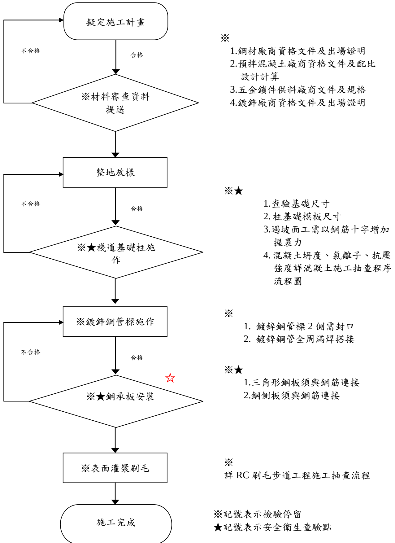
圖 5-16 高架棧道施工檢驗程序
