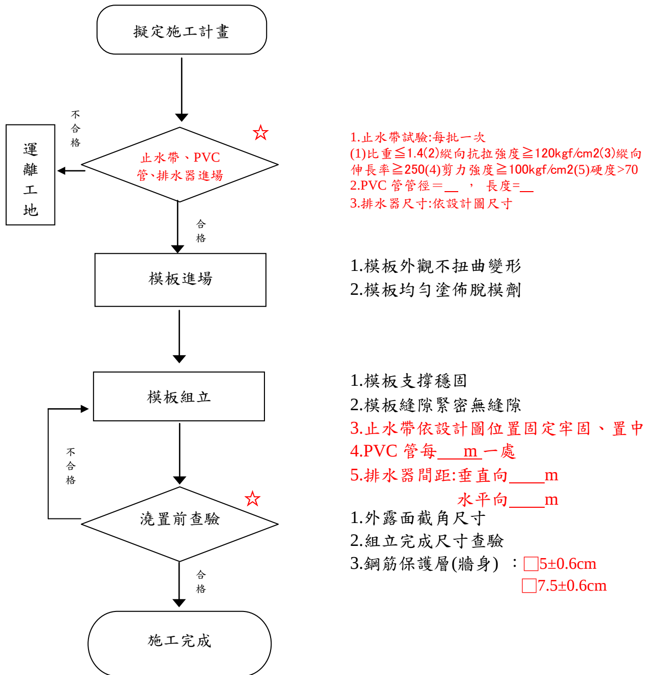
圖三.4 模板工程施工檢驗流程
