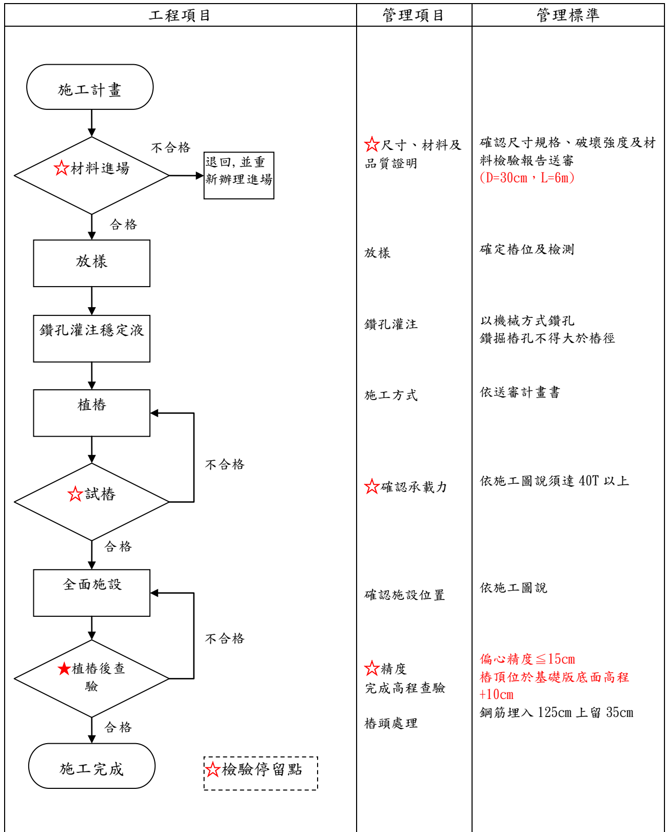
圖 5-22 預力混凝土基樁工程施工檢驗程序
