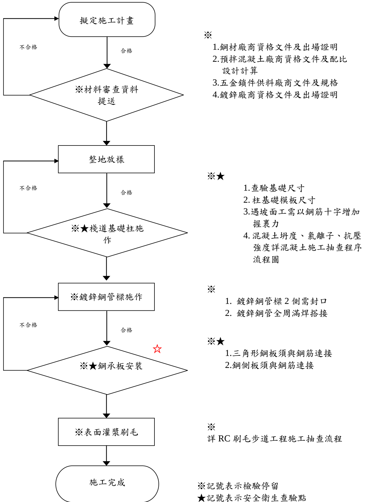
圖 5-17 雙向自行車道施工檢驗程序
