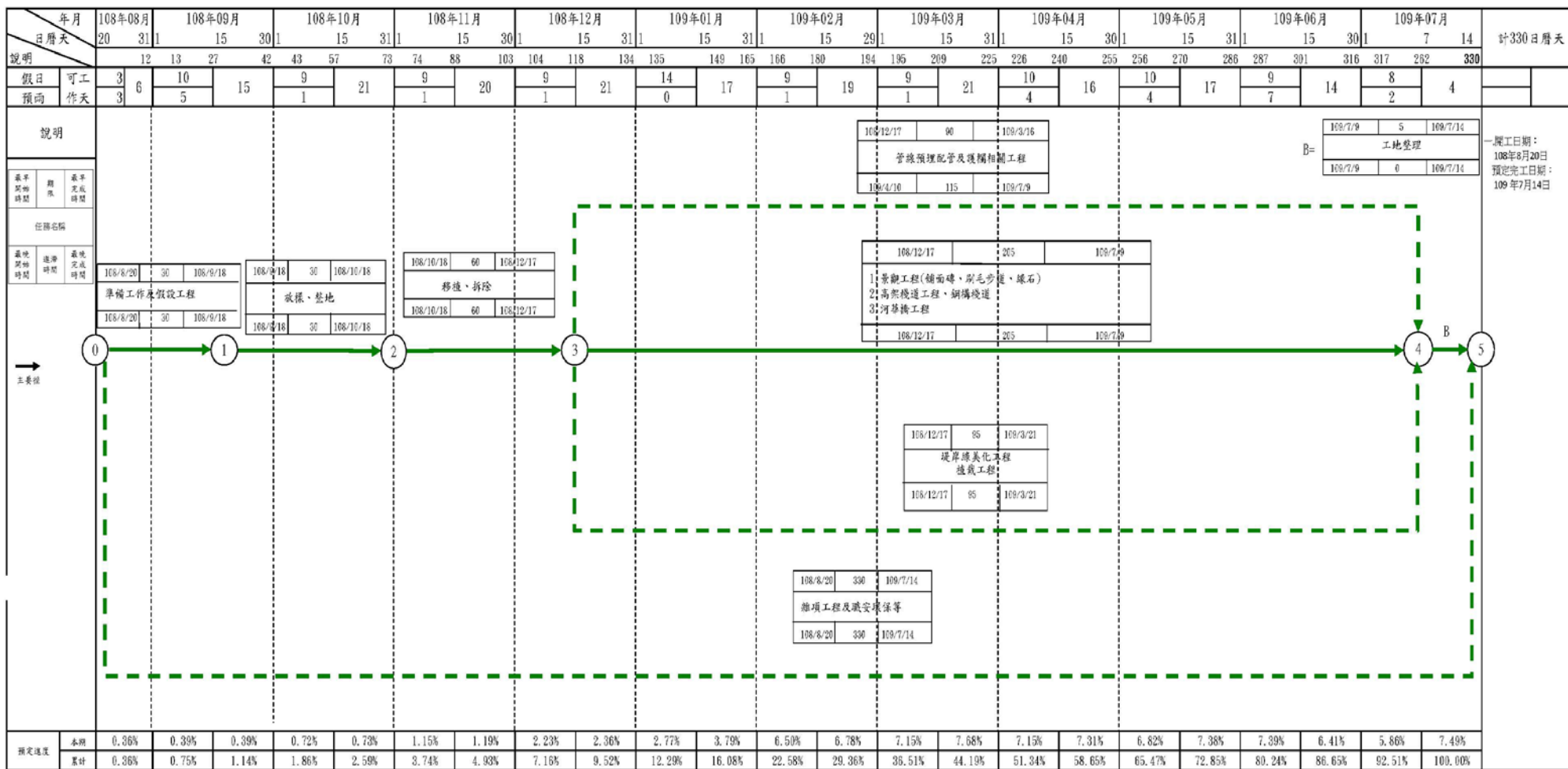
阿公店溪河華橋至高速公路橋水岸環境改善工程---網狀圖
