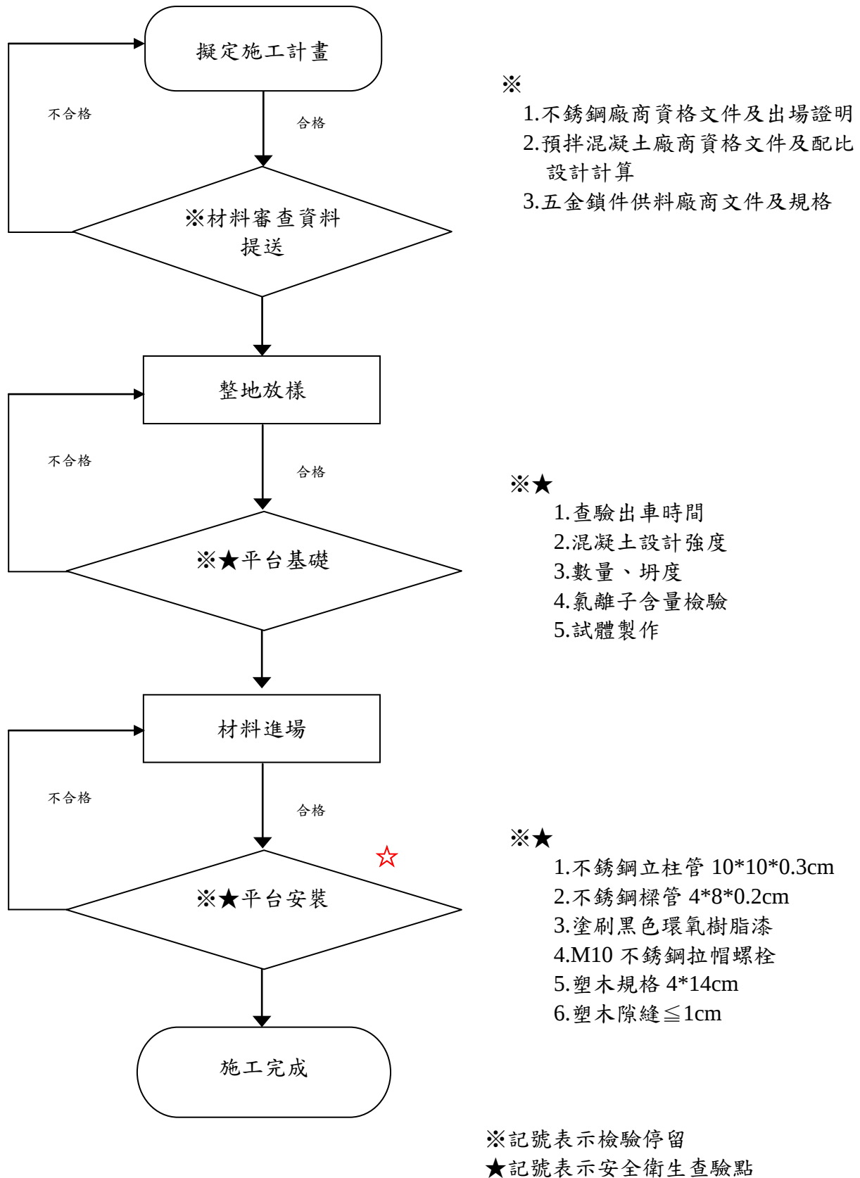
圖 5-18 塑木平台工程施工檢驗程序
