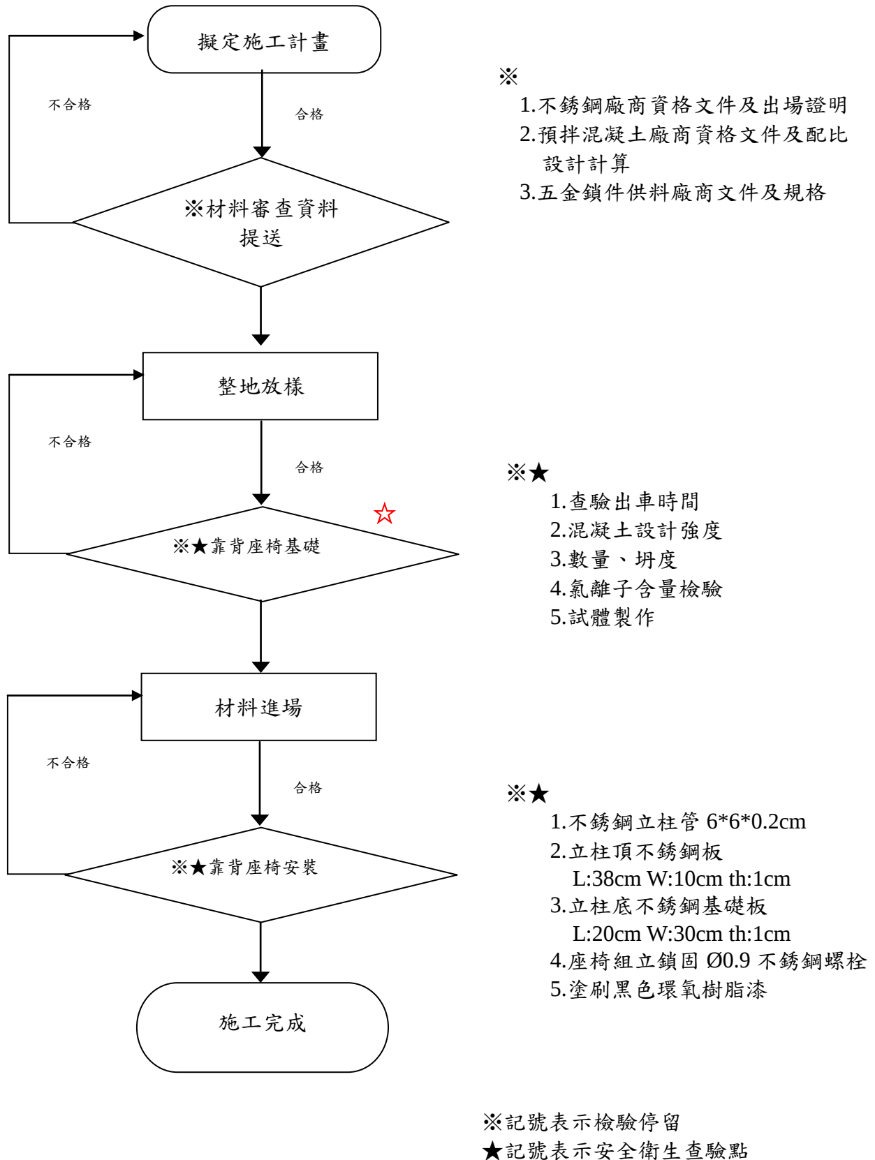
圖三.10 靠背座椅施工檢驗流程
