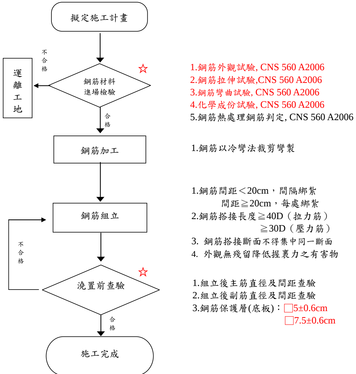
圖三.3 鋼筋工程施工檢驗流程
