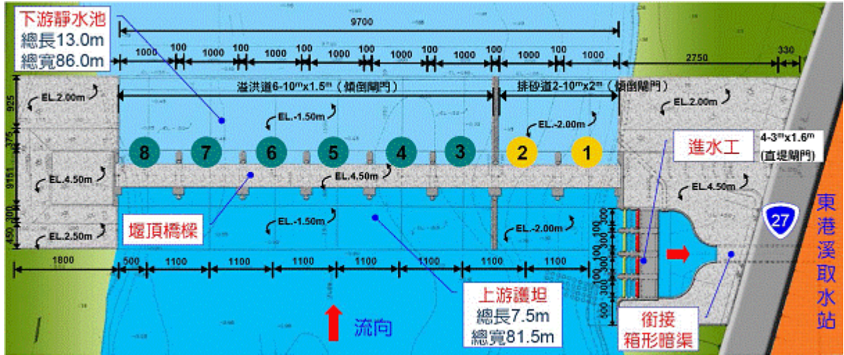
附圖二 東港堰水門布置圖
