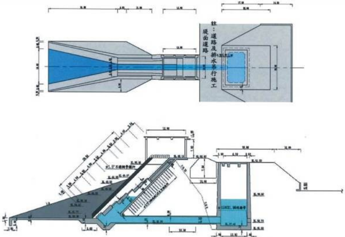
附圖三 取水工水門布置圖
