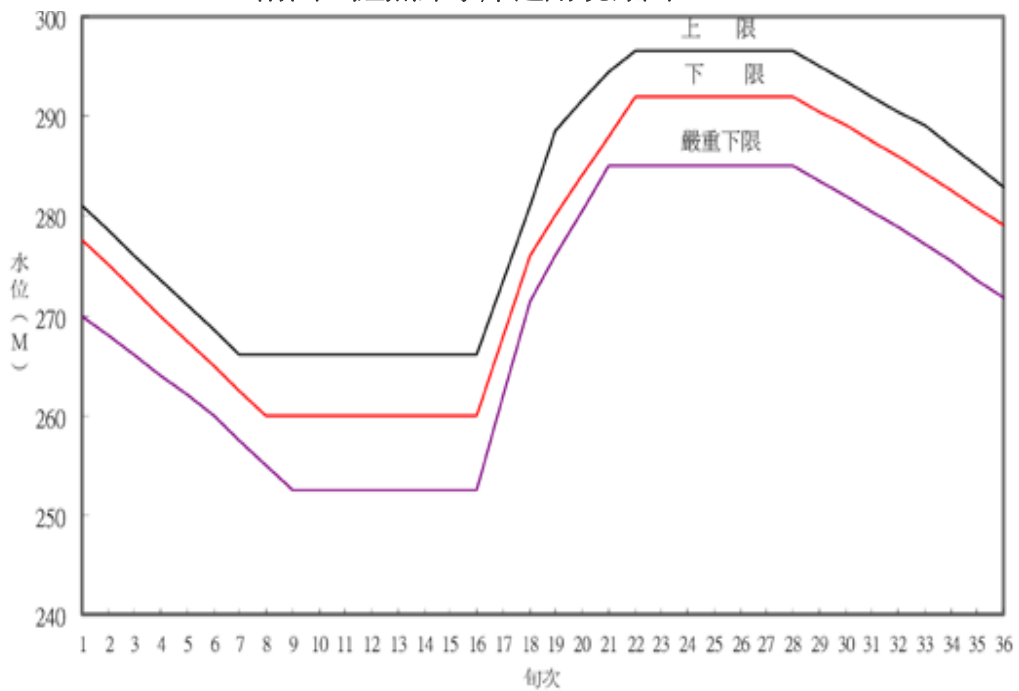
附圖 鯉魚潭水庫運用規線圖
