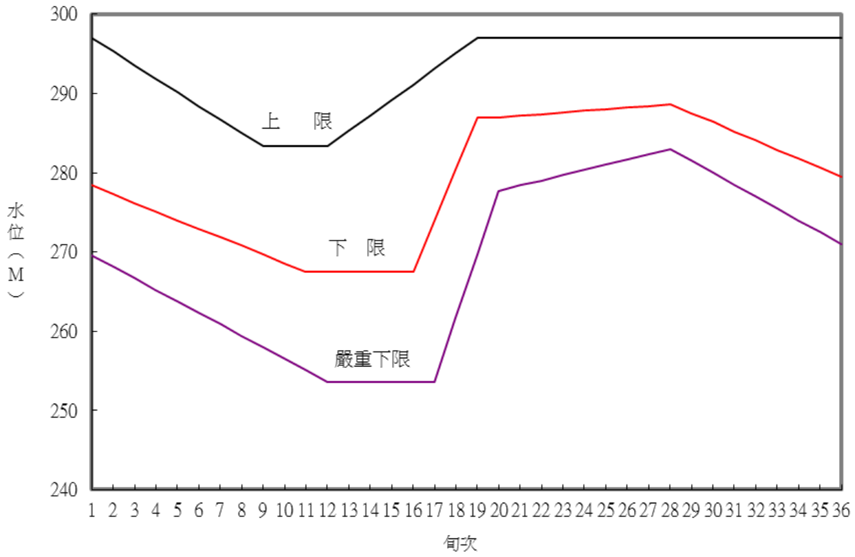
附圖 鯉魚潭水庫運用規線圖
