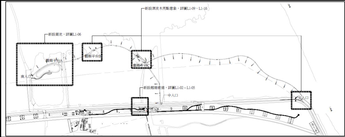
工程平面配置圖
