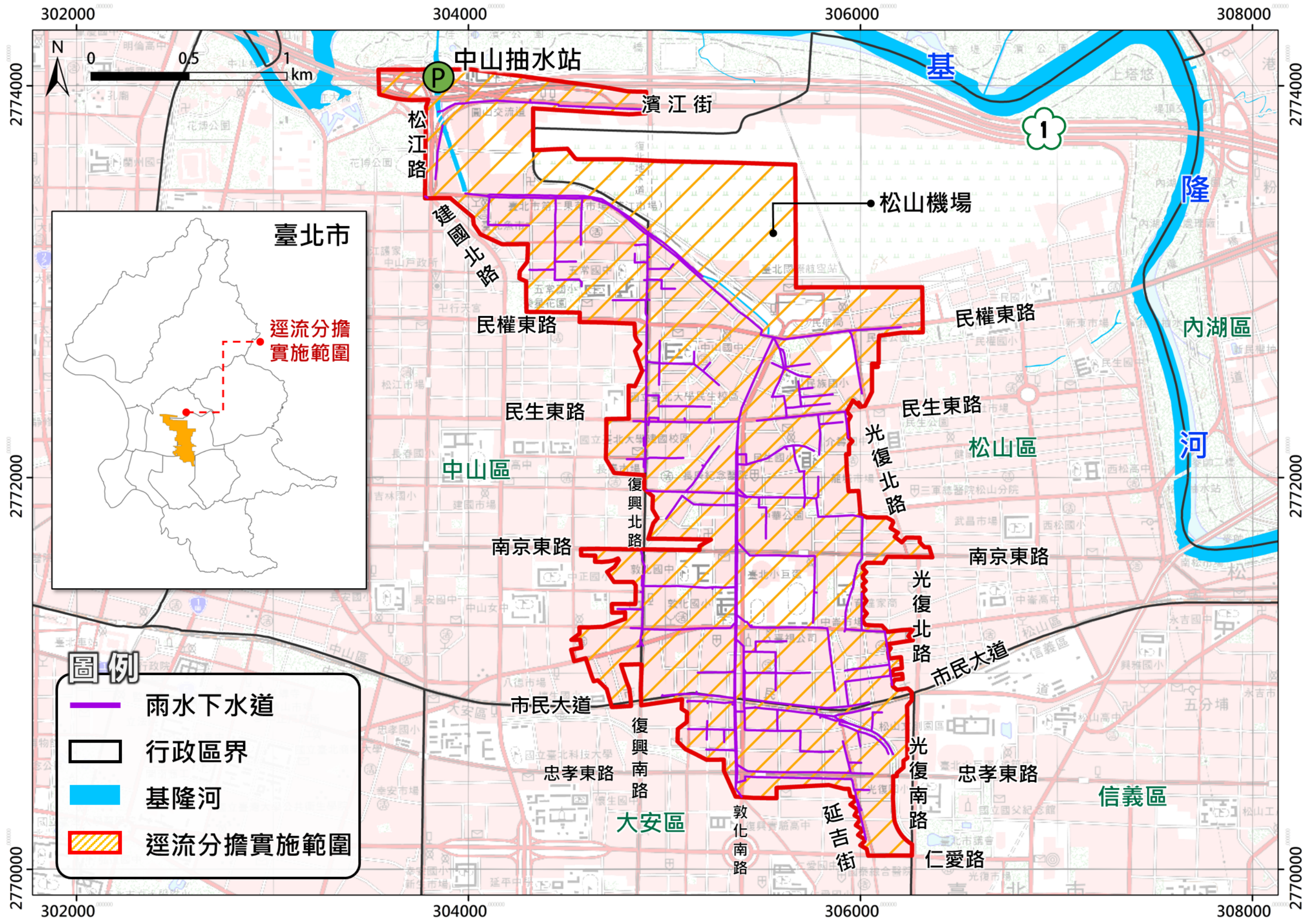
中山抽水站集水分區逕流分擔實施範圍
