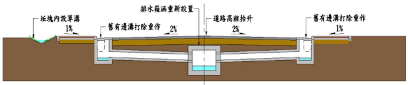
圖 2.1- 19 環港道路改善工程排水改善剖面示意圖
