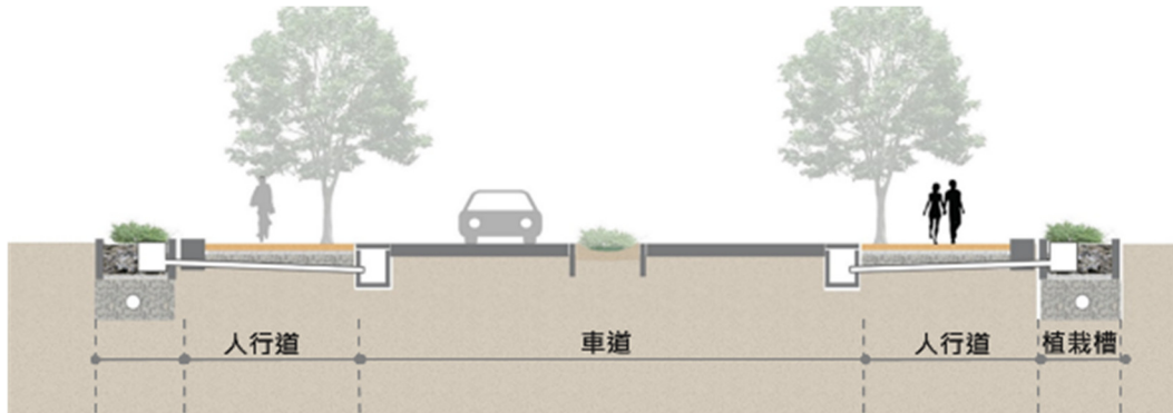
圖 2.1-23 區內道路及排水改善工程—排水改善剖面示意圖
