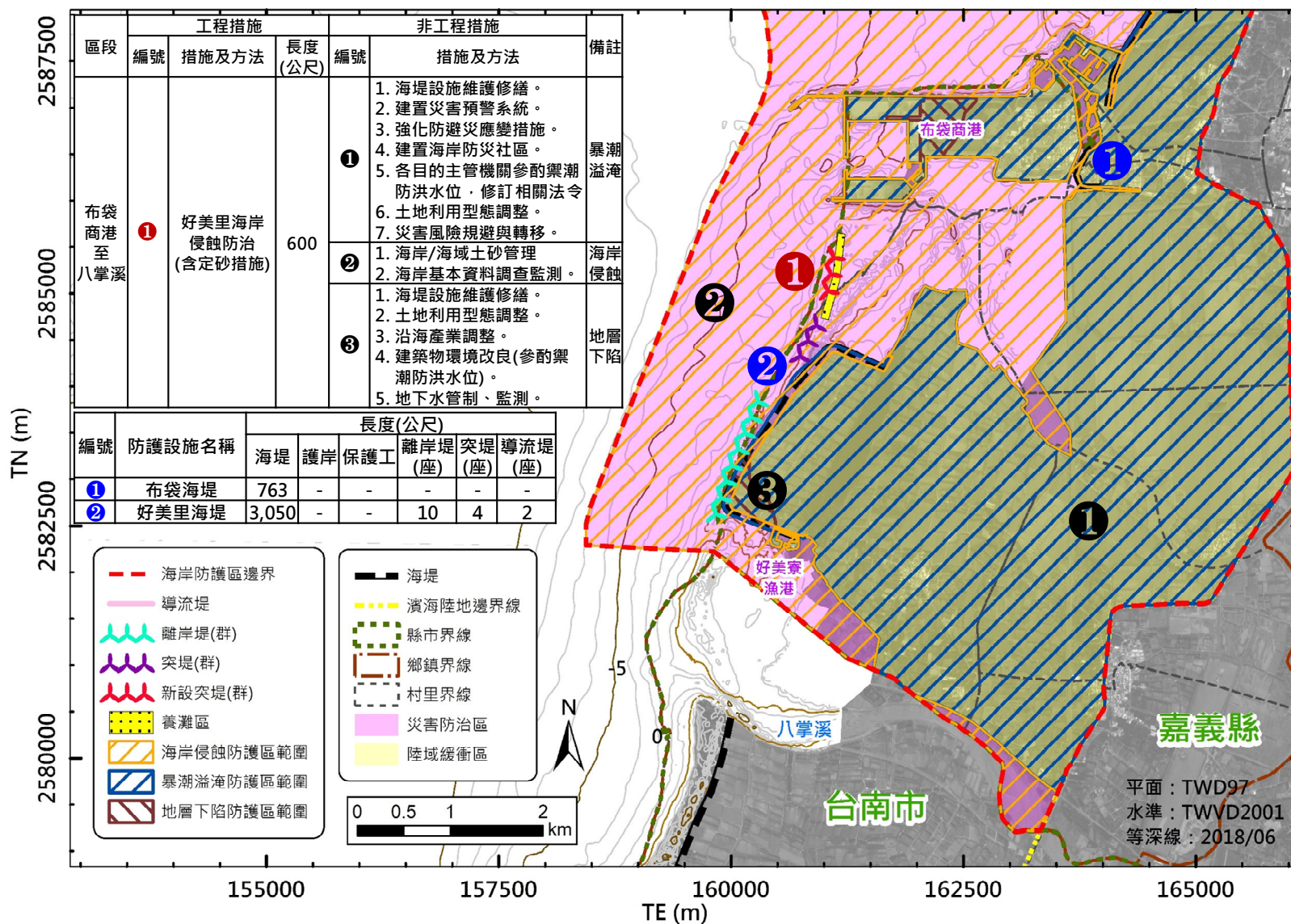
圖7-1 嘉義海岸防護設施種類、規模及配置平面配置圖(3/3)
