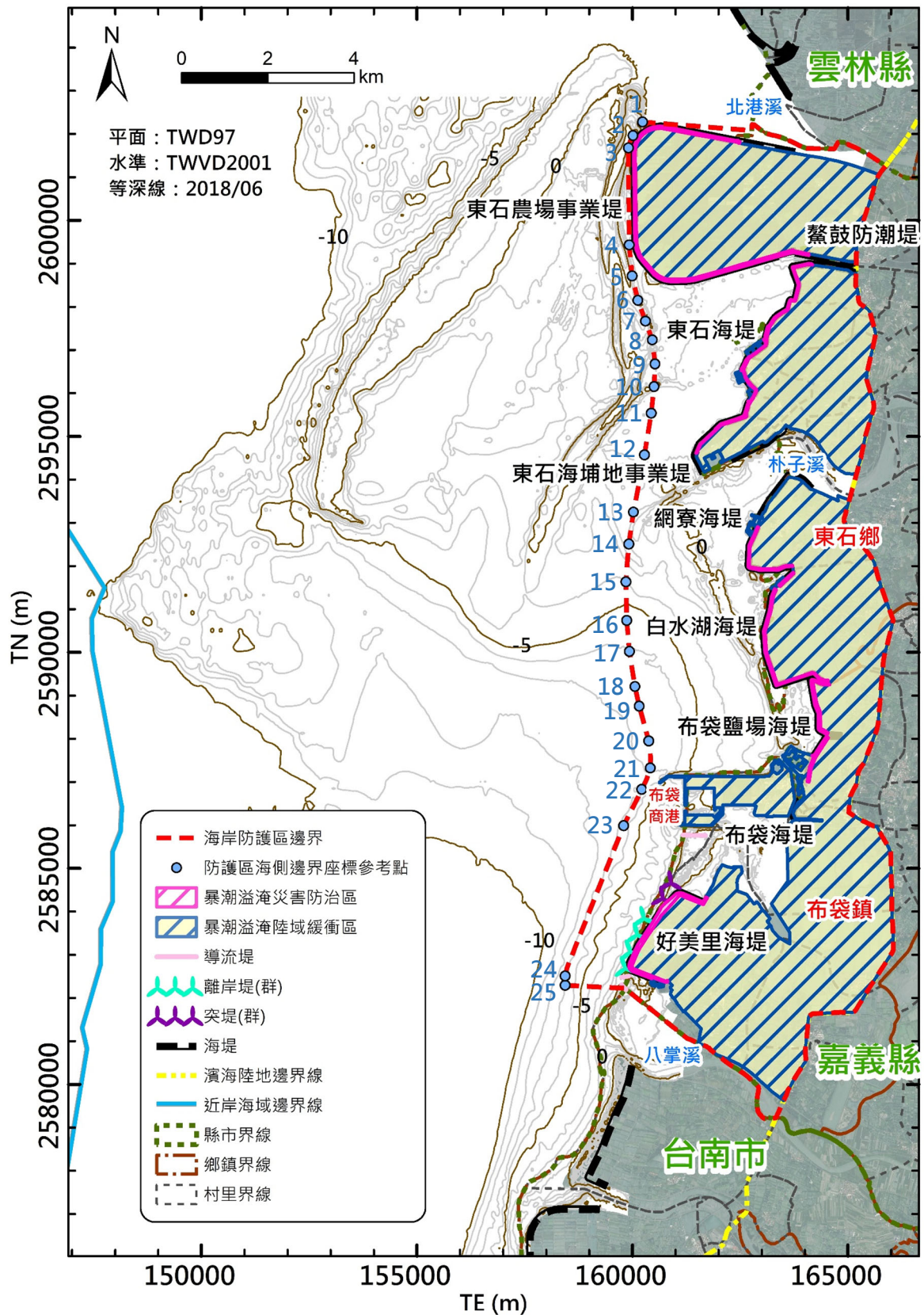
圖4-1 嘉義縣一級海岸防護區暴潮溢淹災害防治區與陸域緩衝區範圍圖
