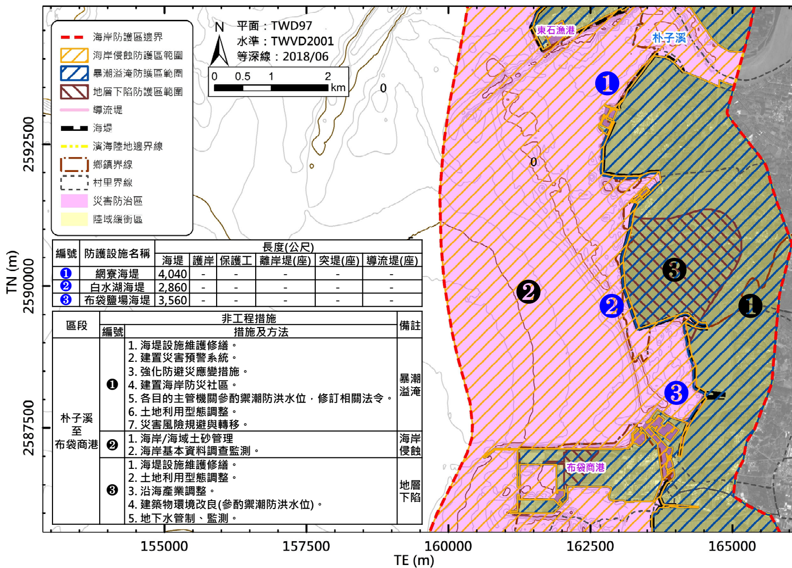
圖7-1 嘉義海岸防護設施種類、規模及配置平面配置圖(2/3)
