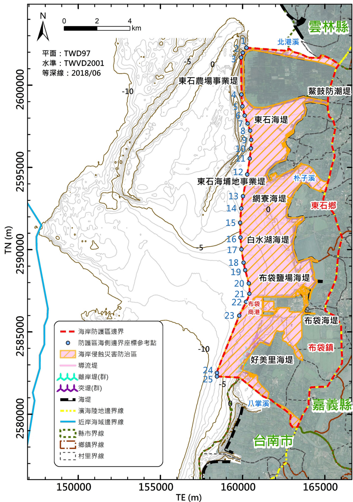
圖4-2 嘉義縣一級海岸防護區海岸侵蝕災害防治區範圍圖
