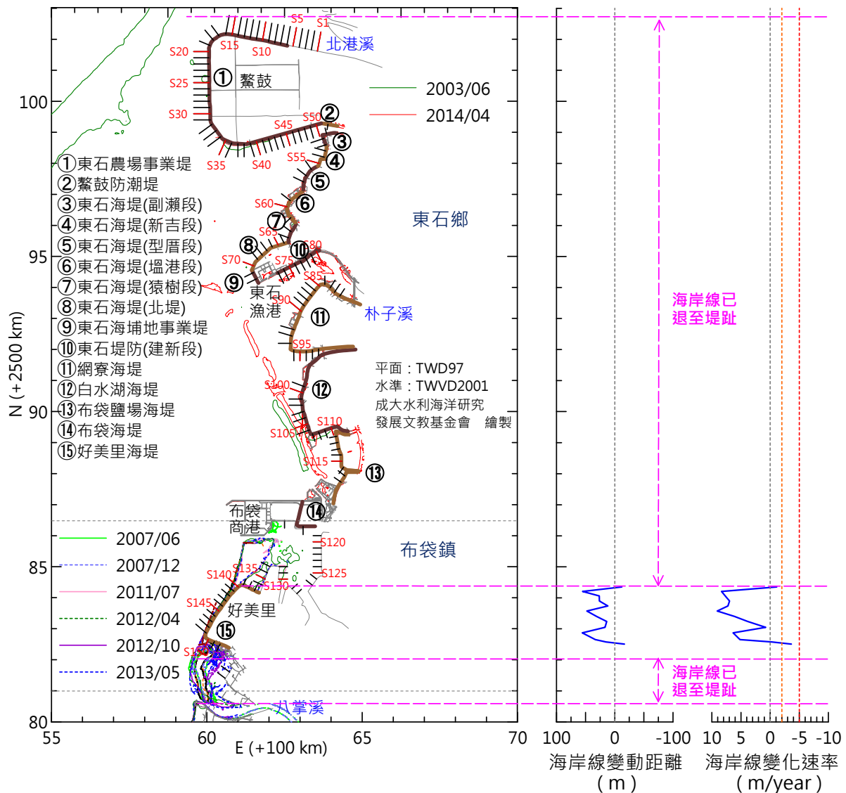
圖2-8 嘉義海岸侵蝕潛勢圖(斷面變動距離及變化速率)
