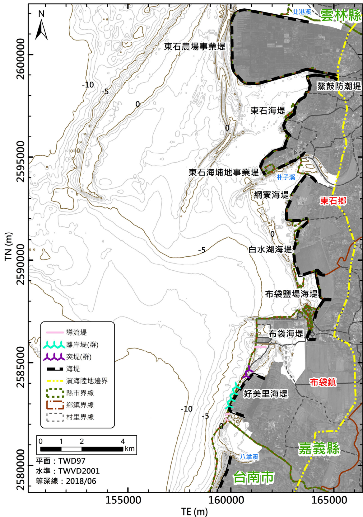
圖2-4 海岸防護設施分佈圖
