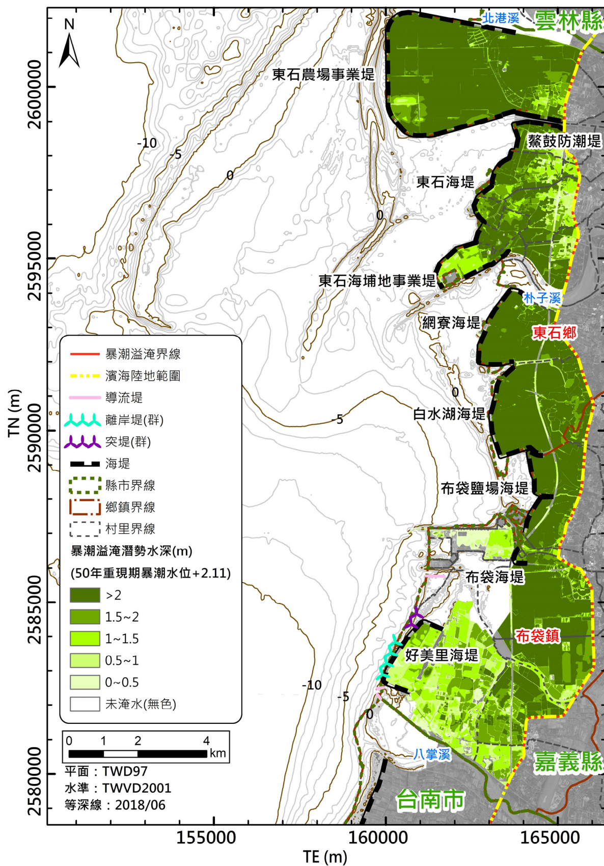
圖2-6 嘉義縣一級海岸50年重現期暴潮溢淹潛勢(潛勢水深)範圍圖
