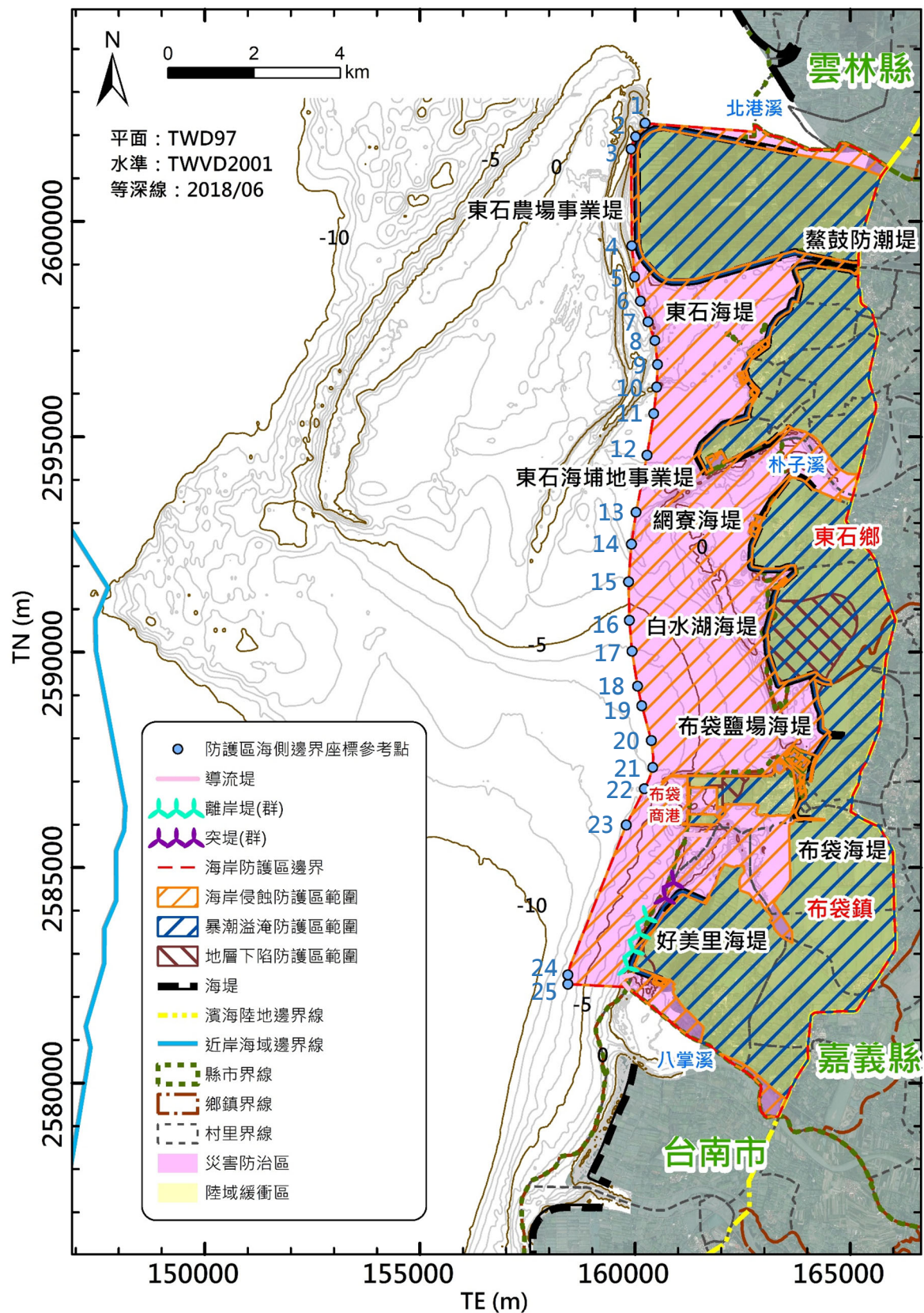
圖4-4 嘉義縣一級海岸防護區範圍圖
