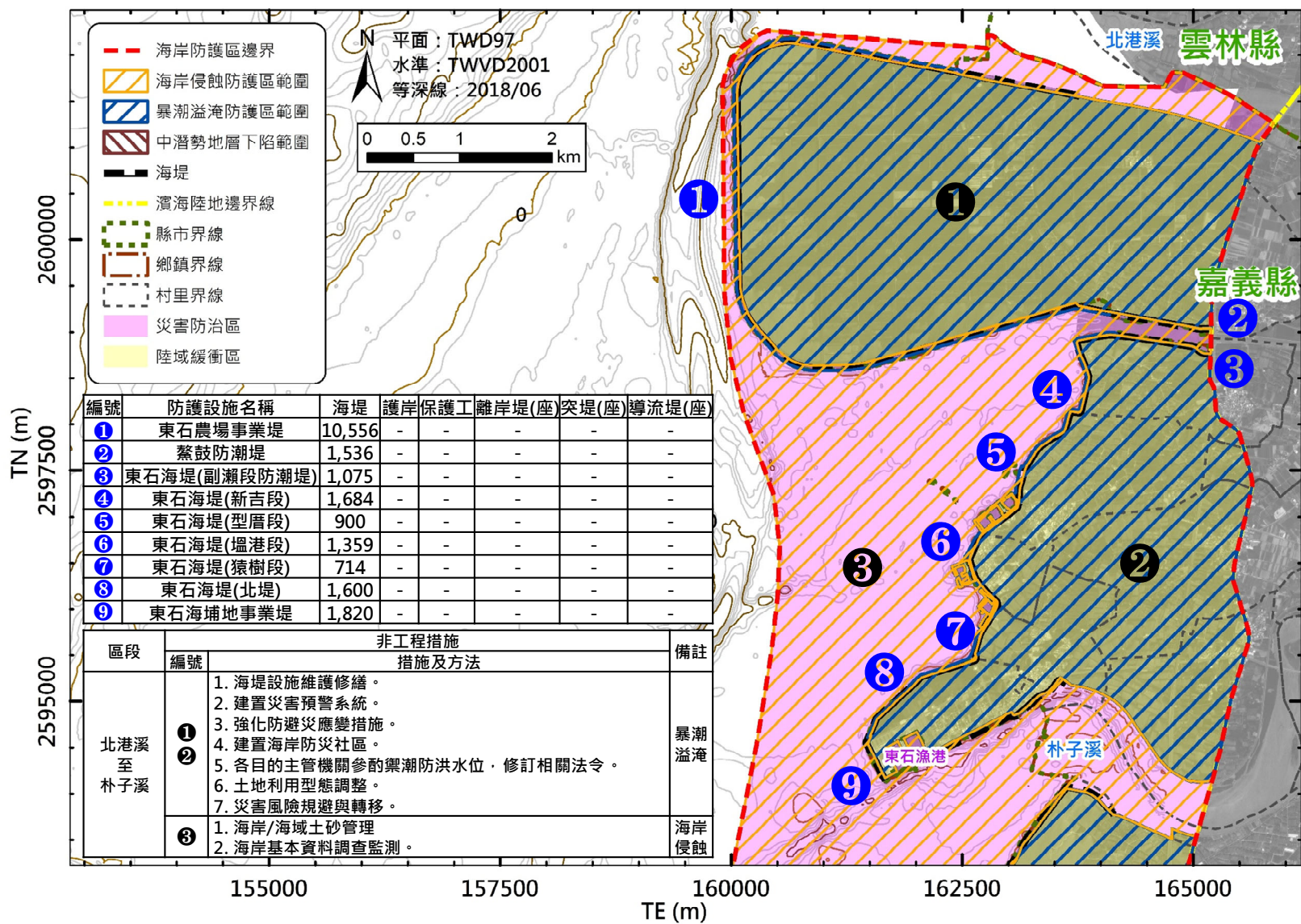
圖7-1 嘉義海岸防護設施種類、規模及配置平面配置圖(1/3)
