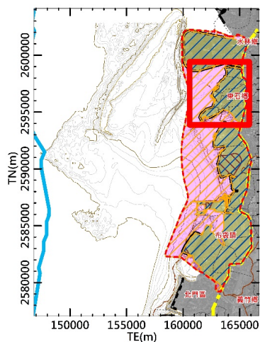
嘉義縣一級海岸防護區範圍圖(六腳大排水溝-朴子溪)
