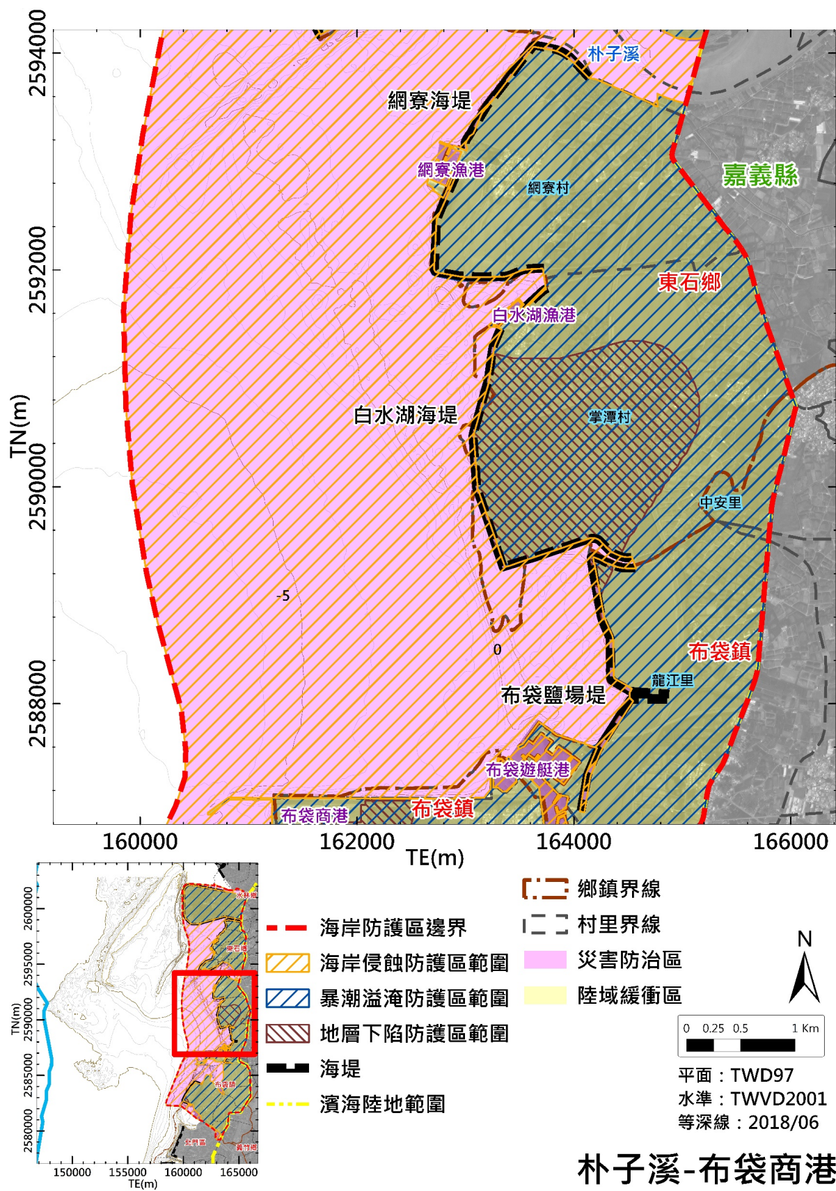
嘉義縣一級海岸防護區範圍圖(朴子溪-布袋商港)
