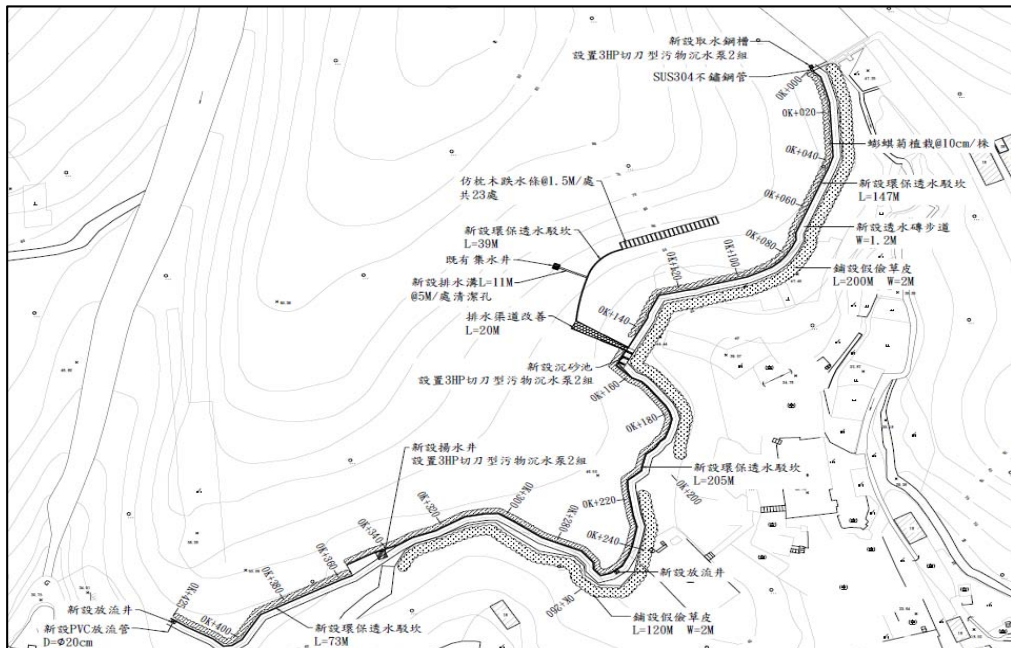
圖 18 基地「水庫周邊設施」規劃平面配置圖
