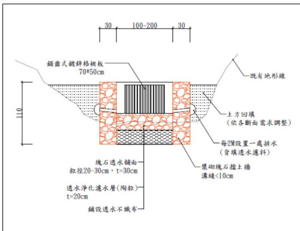
圖 20 基地「排水渠道改善」斷面詳圖
