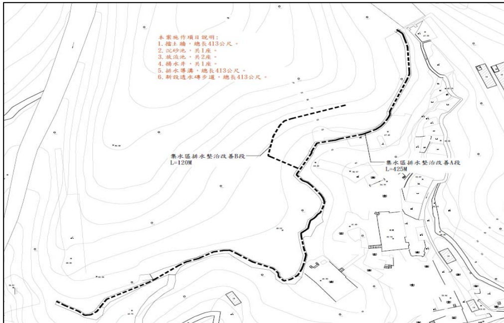
圖 17 基地「排水整治改善」規劃平面配置圖
