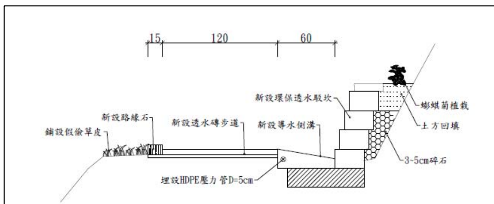
圖 19 基地「上游排水路段」規劃斷面圖
