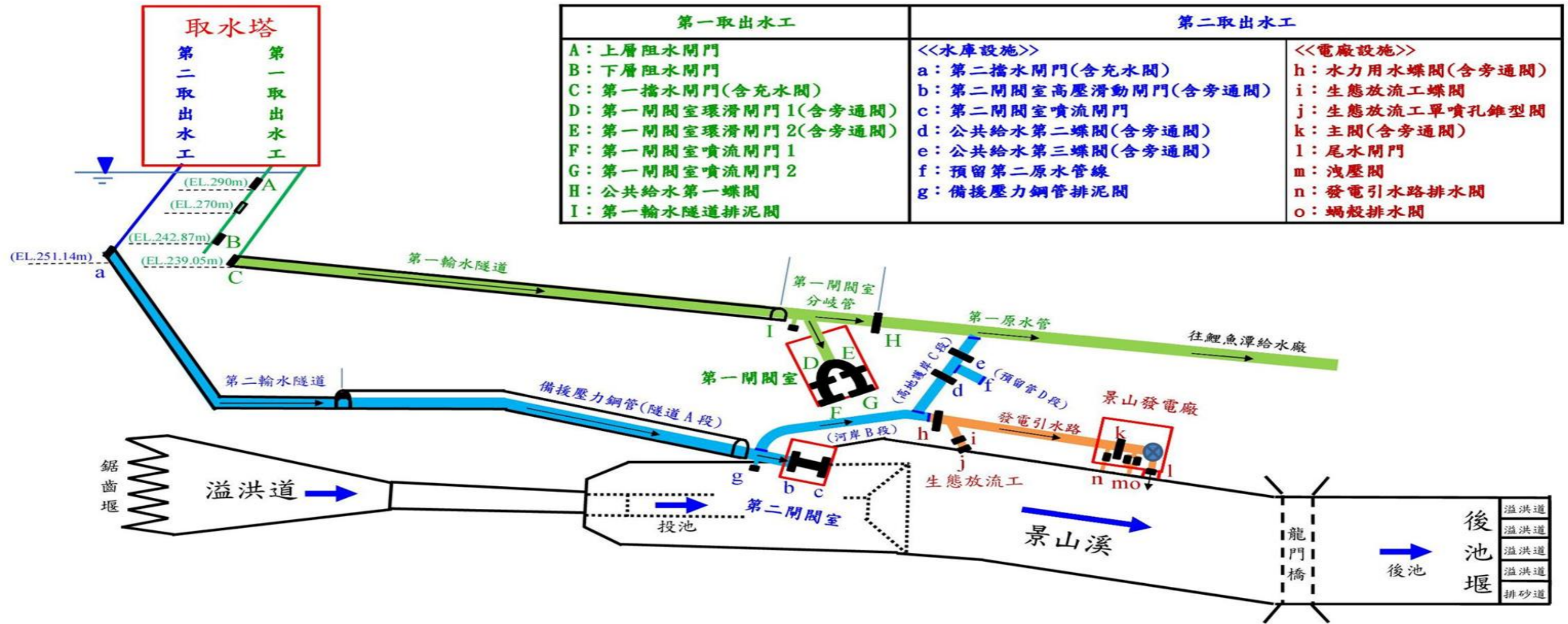
附圖、鯉魚潭水庫主要設施圖
