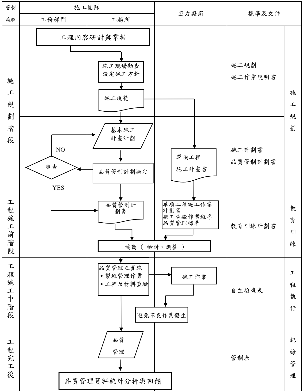
圖 2- 2 工地品質管制作業流程
